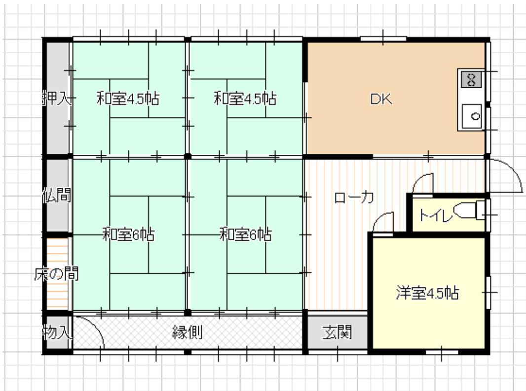
間取図
