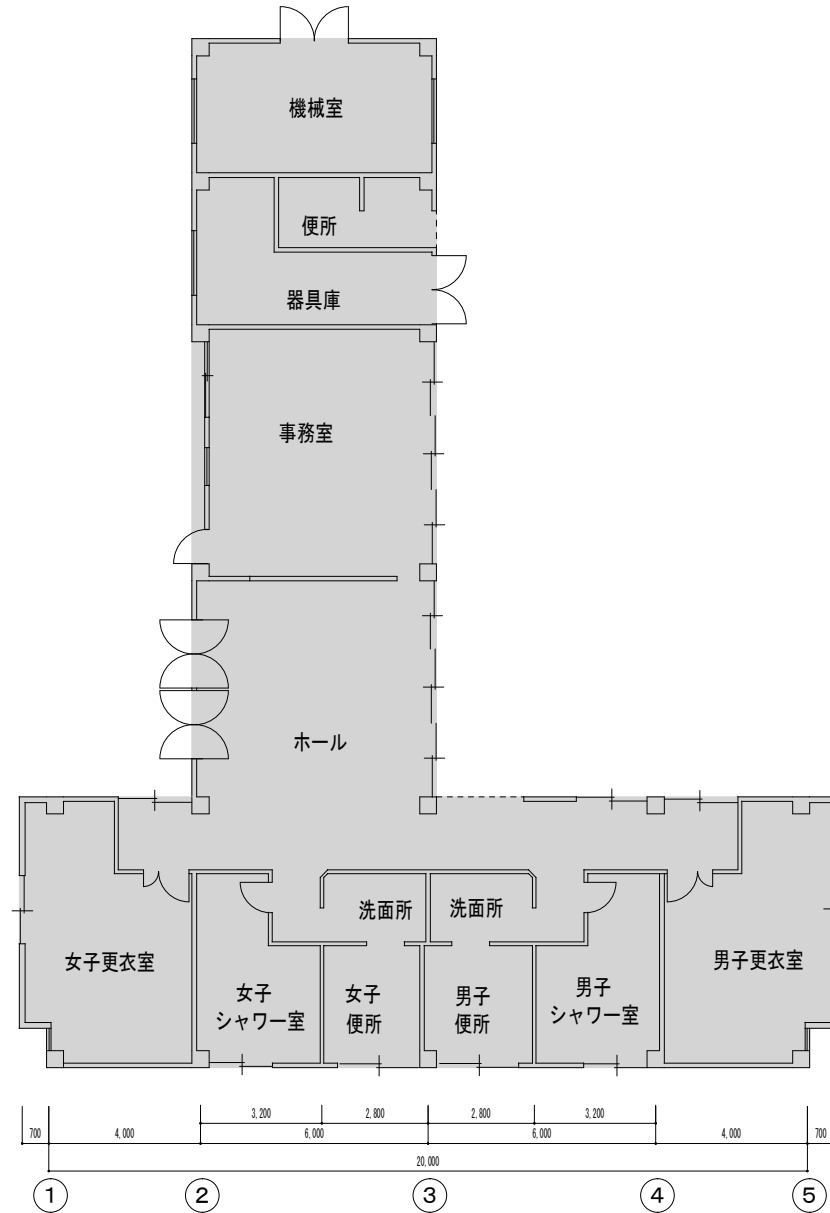
1 階平面図
