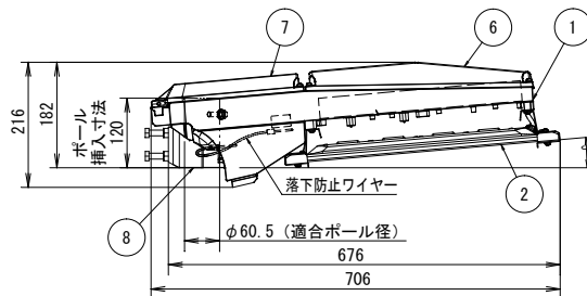
灯具詳細図
