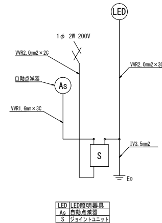
ホール内結線図
