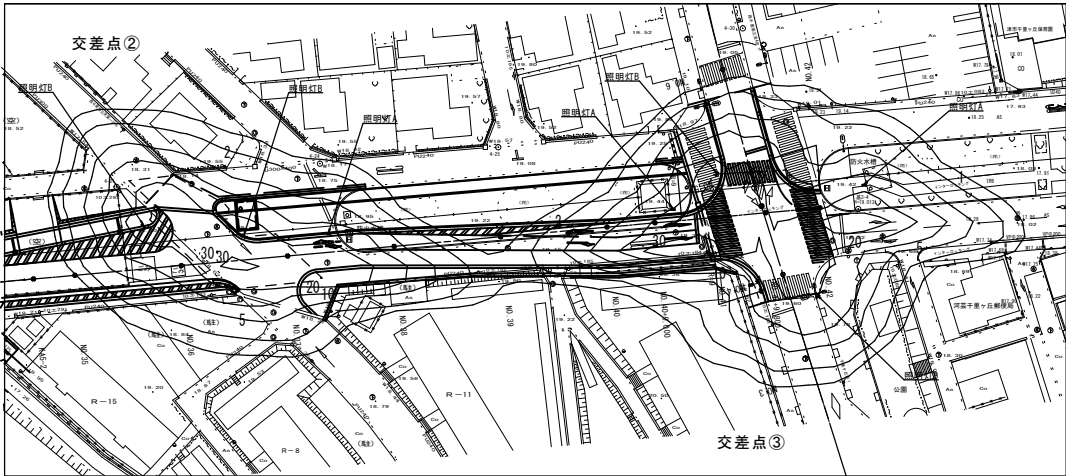
照度分布図
