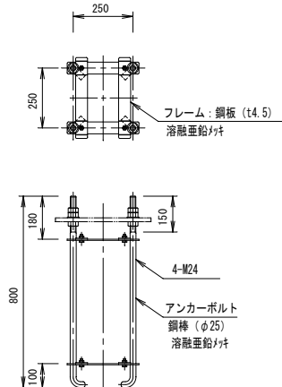
アンカーフレーム詳細図
