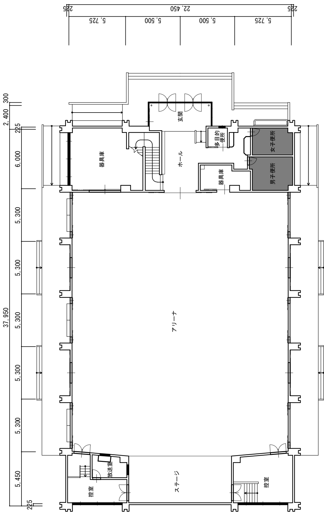
1 階平面図
