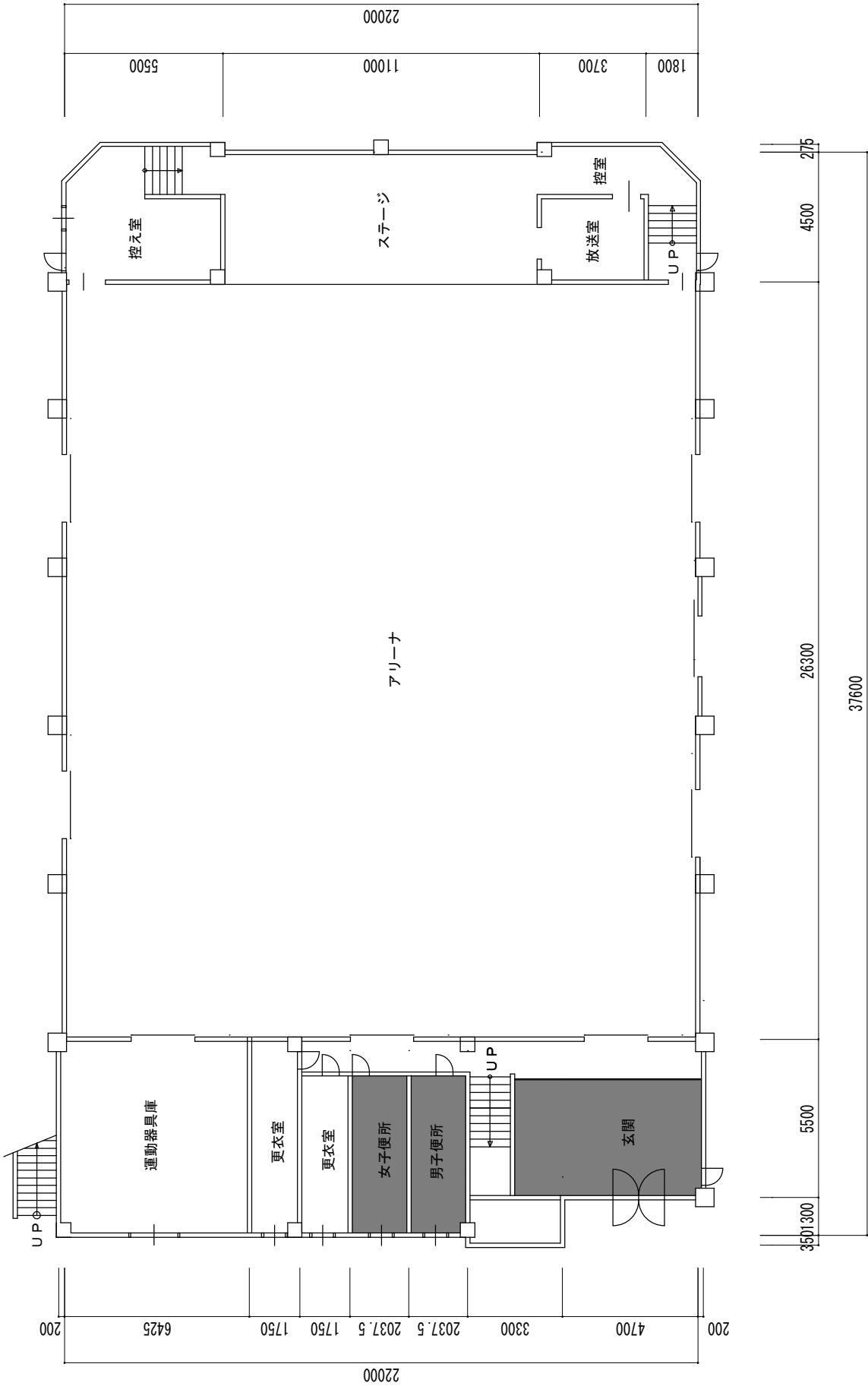
1 階平面図
