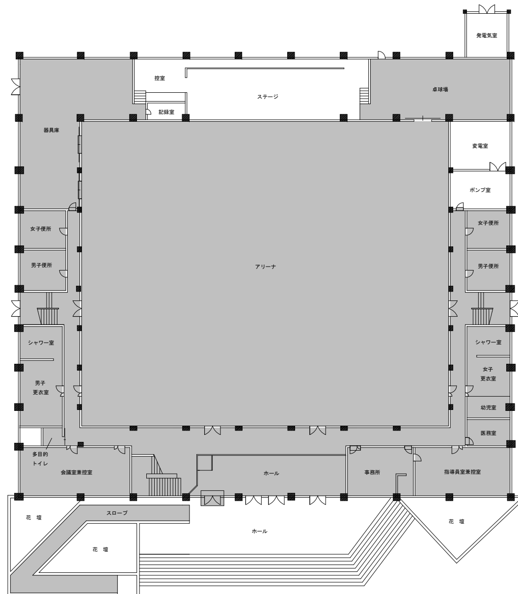
1階平面図
