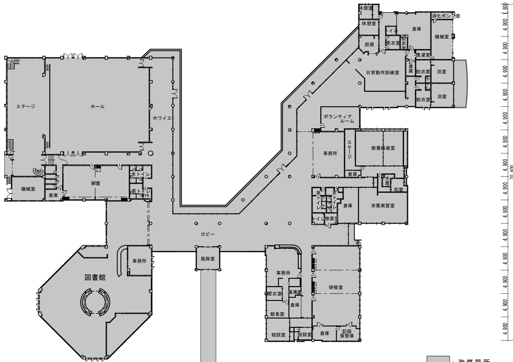
1 階平面図
