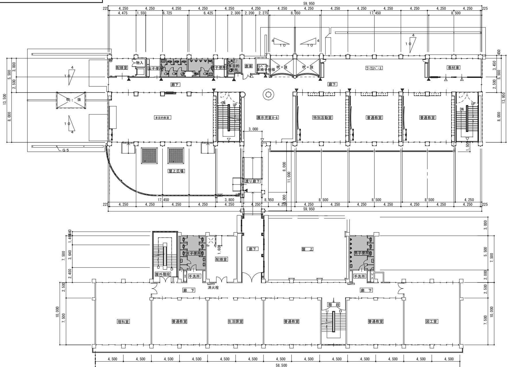
2階平面図
