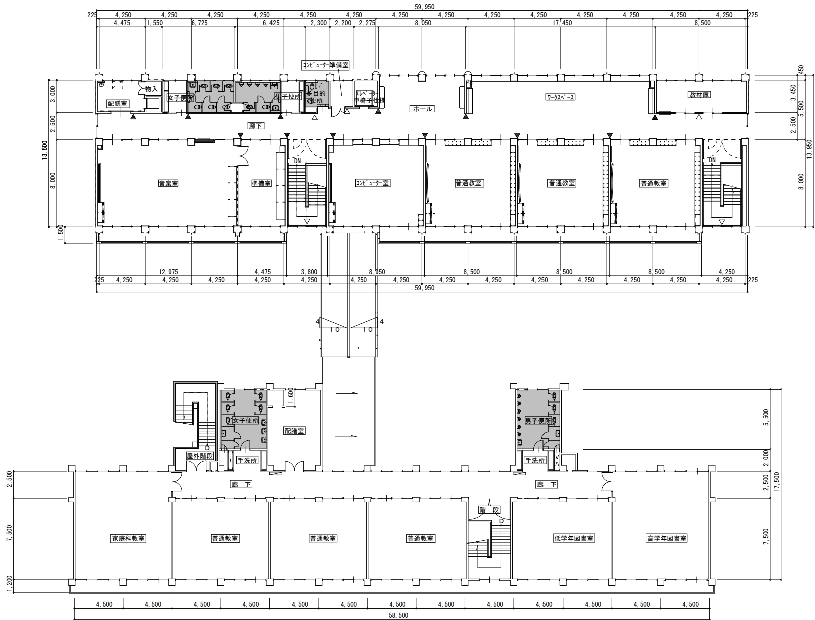
3階平面図
