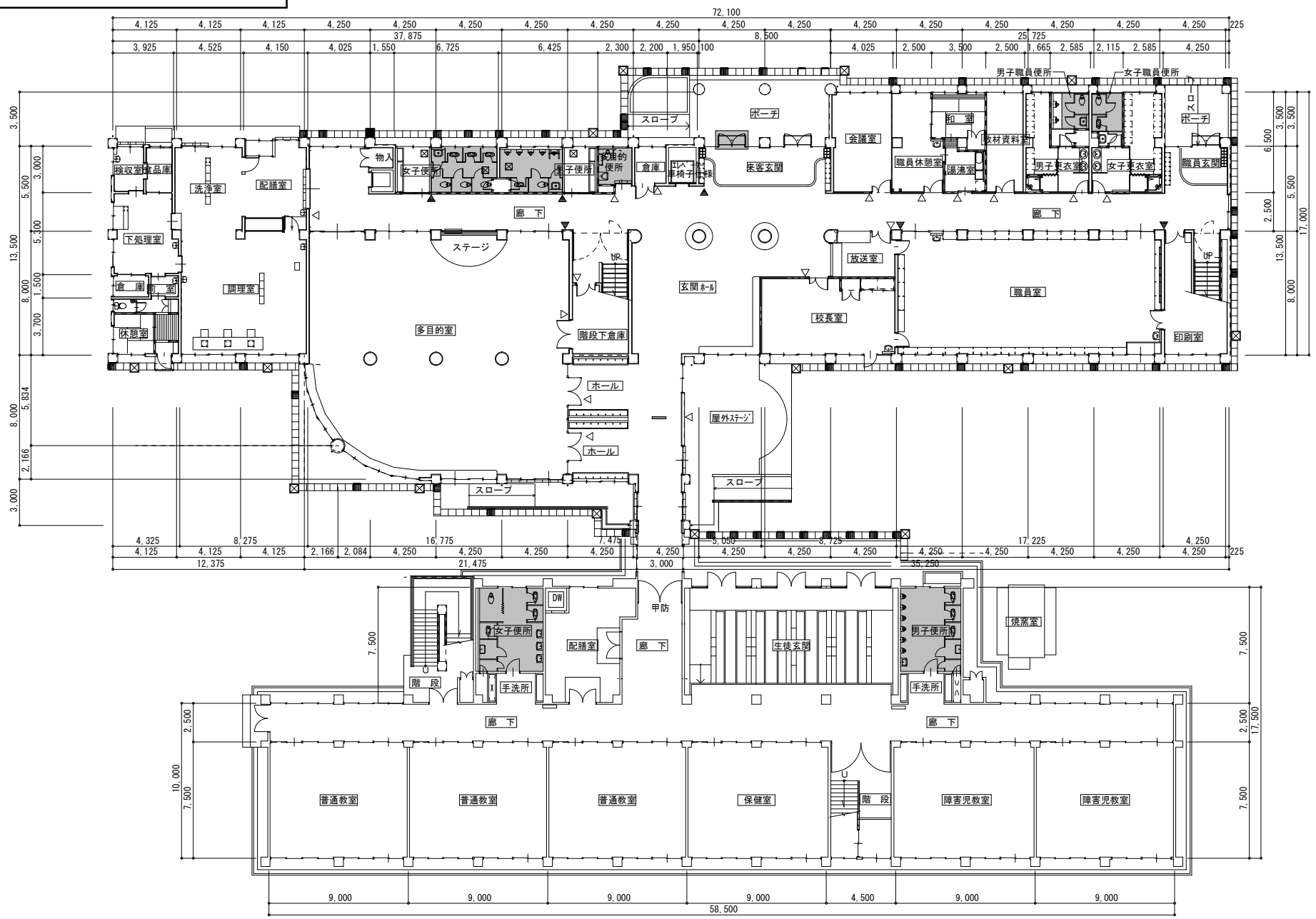
1階平面図
