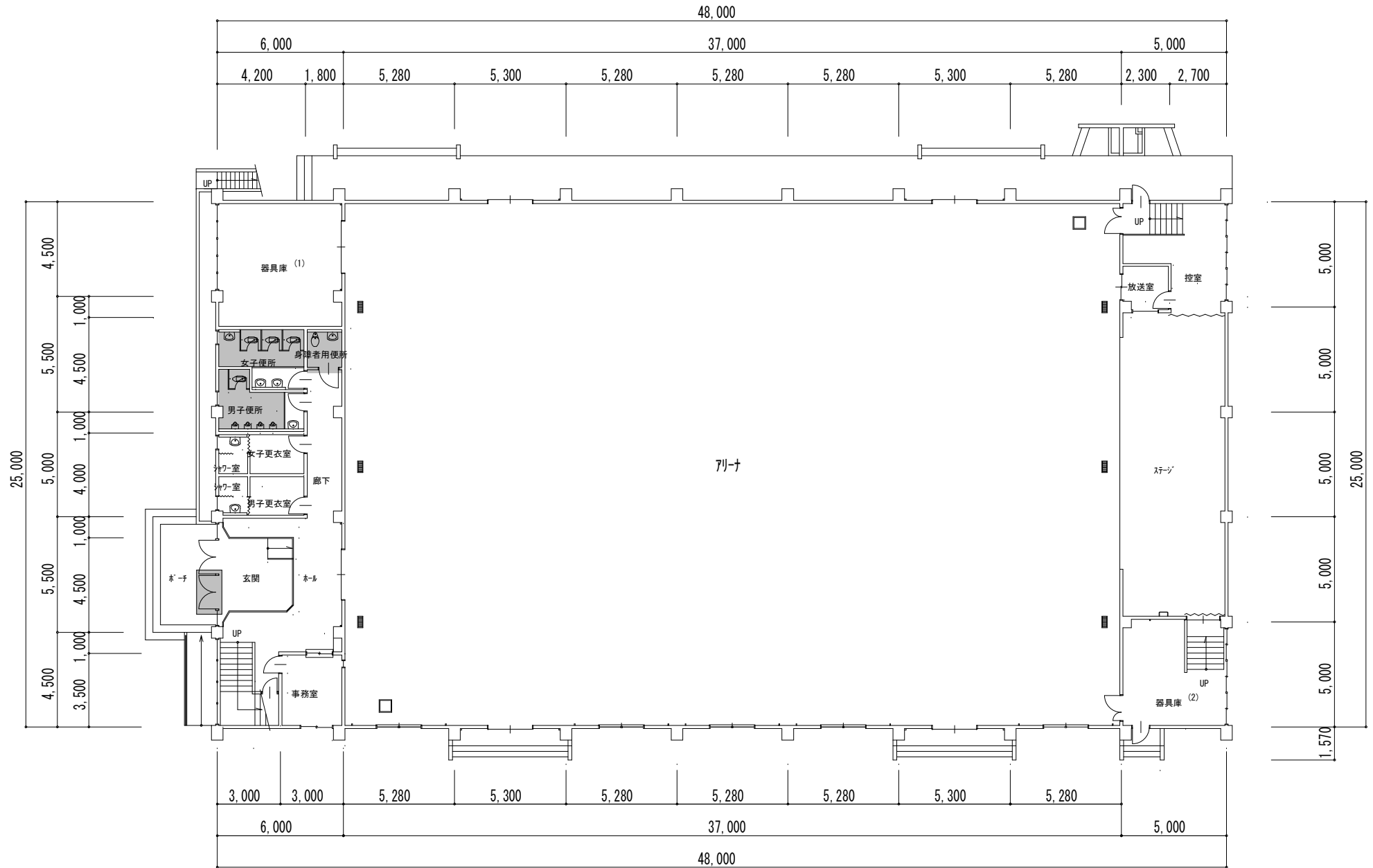
1階平面図
