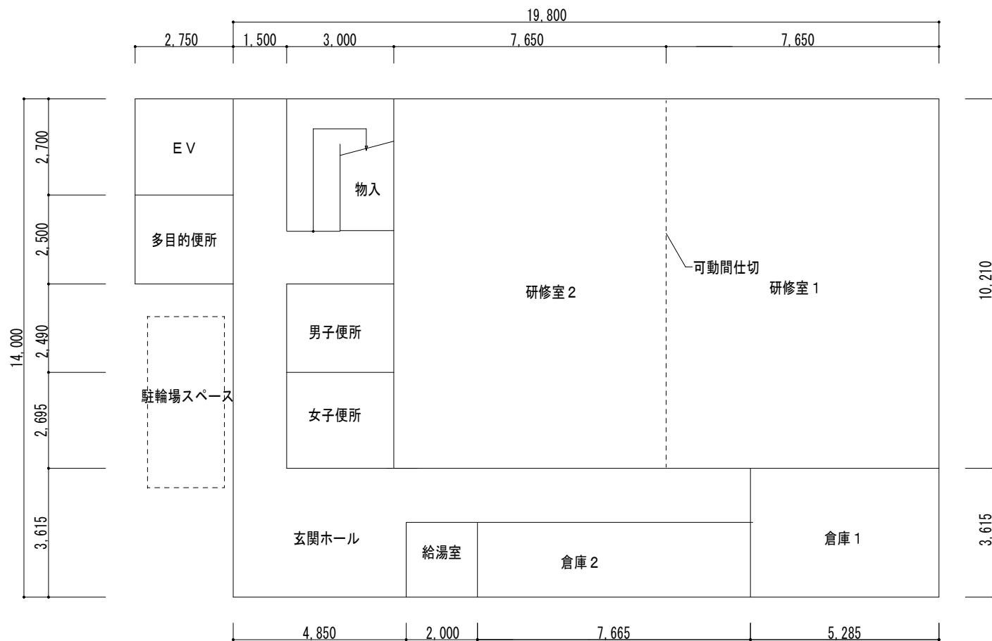
1 階平面図 (参考)
