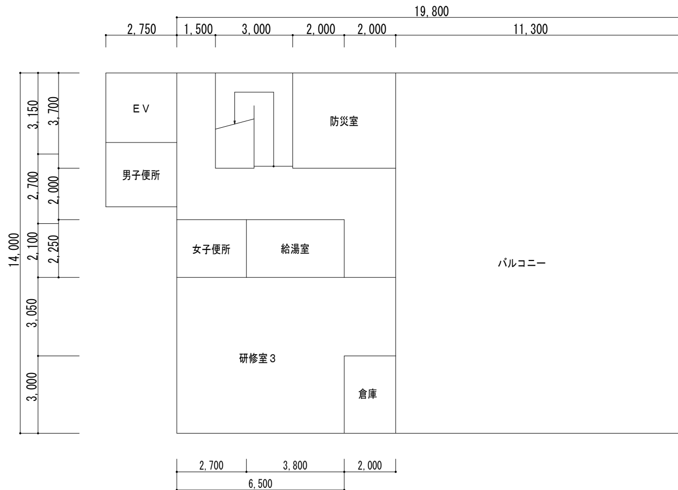
2階平面図(参考)
