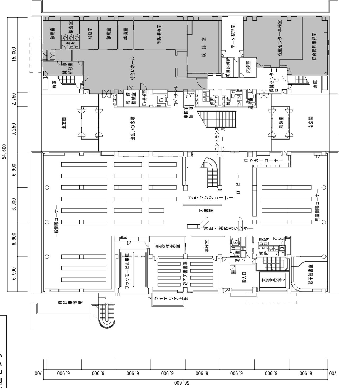
1階平面図
