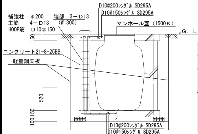
浄化槽断面図 1/50
