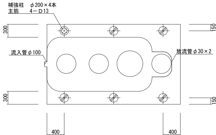
浄化槽平面図 1/50
