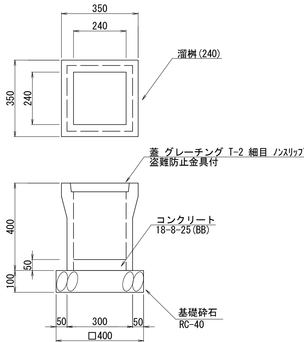
プレキャスト集水樹 S=1:20
