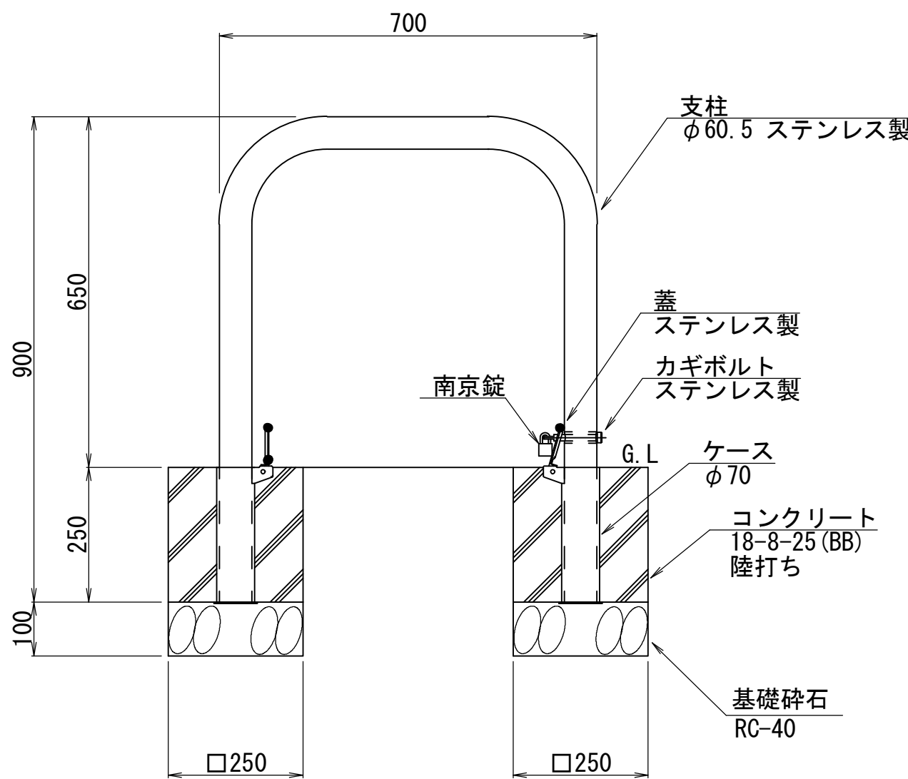
車止め S=1:20
