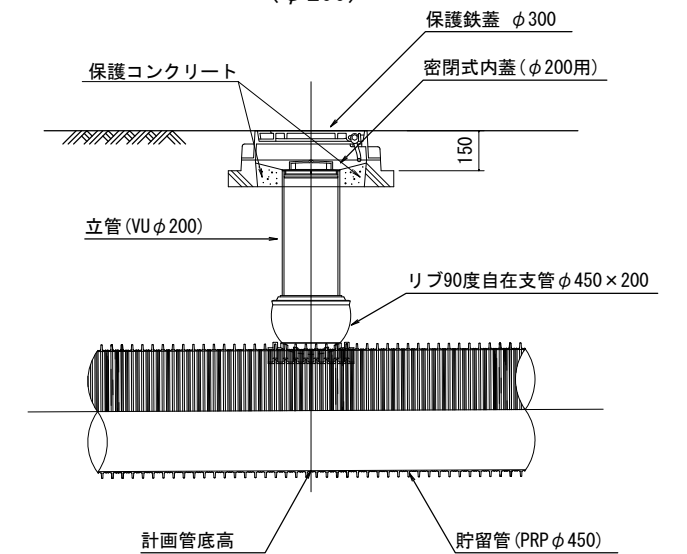
MT3～MT5・注水用マンホール (φ200)
