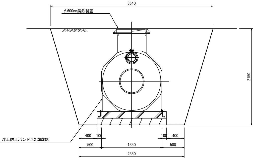
正面図
