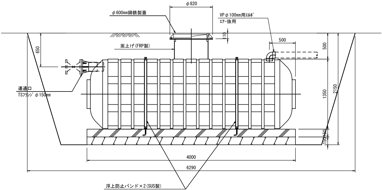
側面図
