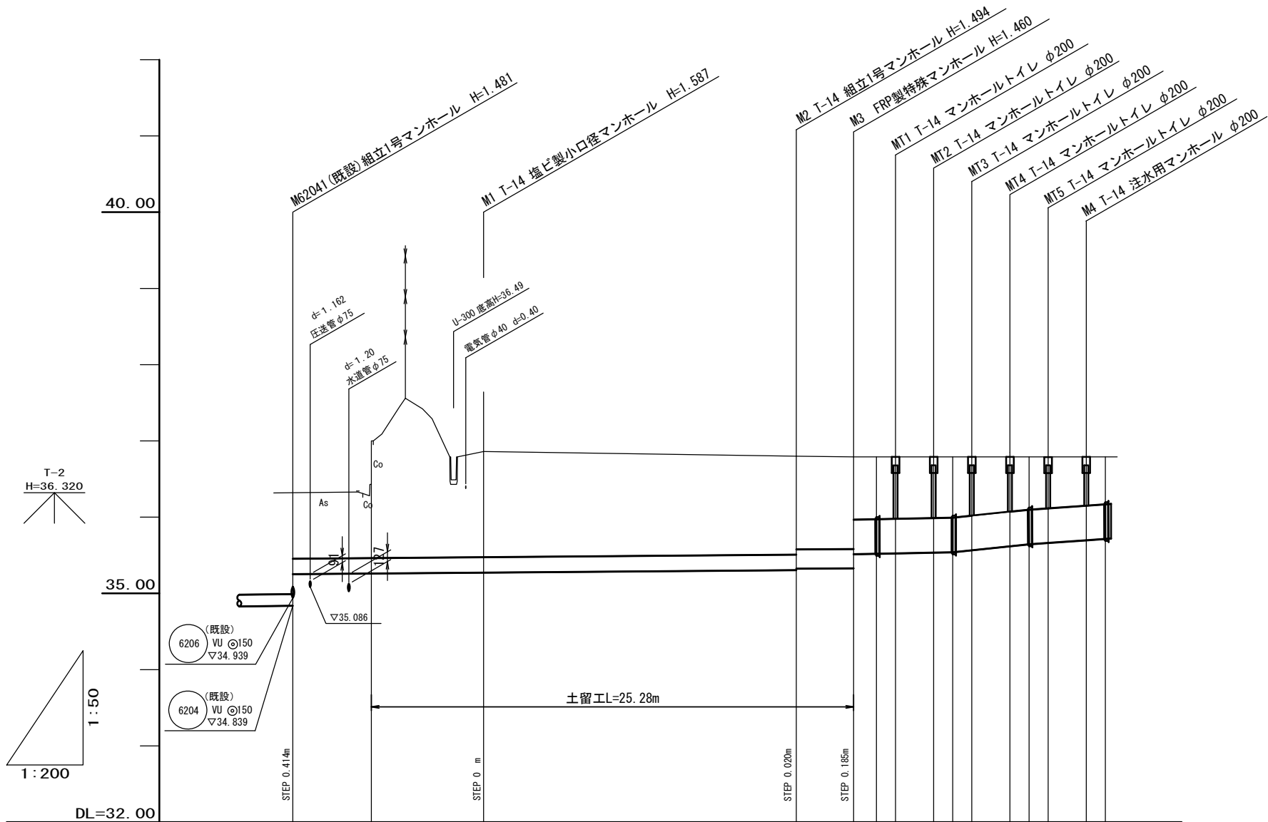
縦断面図 V=1: 50 H=1: 200
