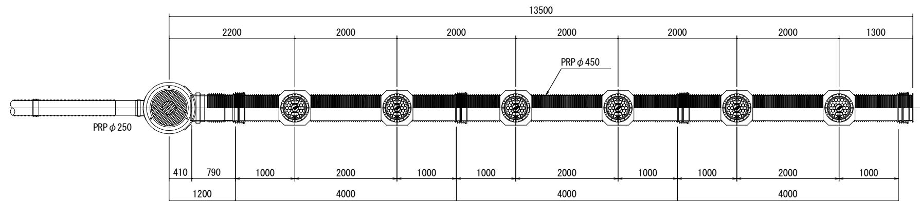
平面図 S=1:50
