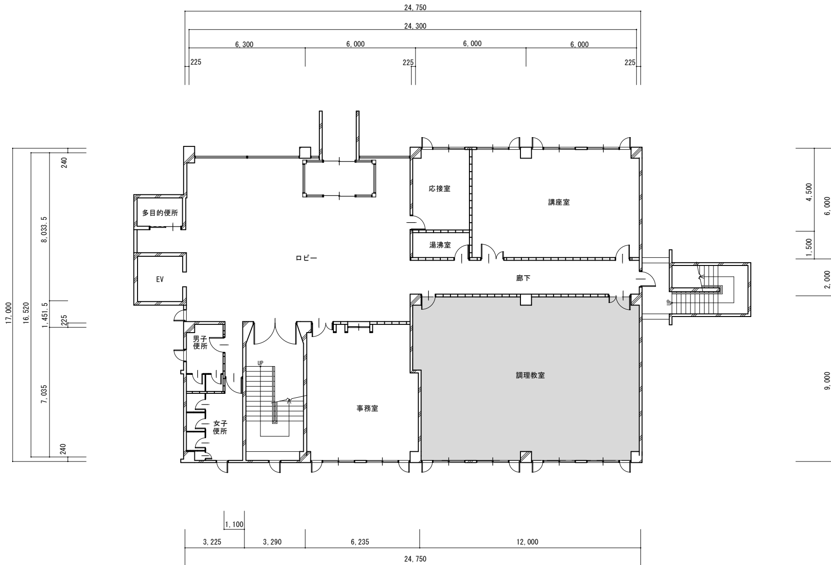
1階平面図
