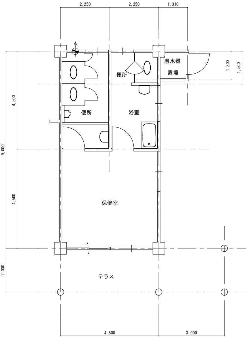
1階平面図
