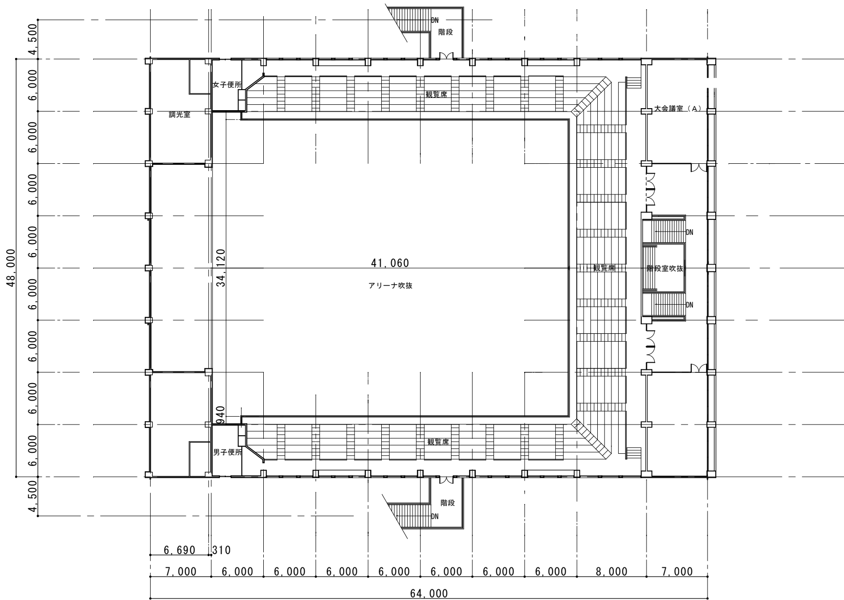
2階平面図
