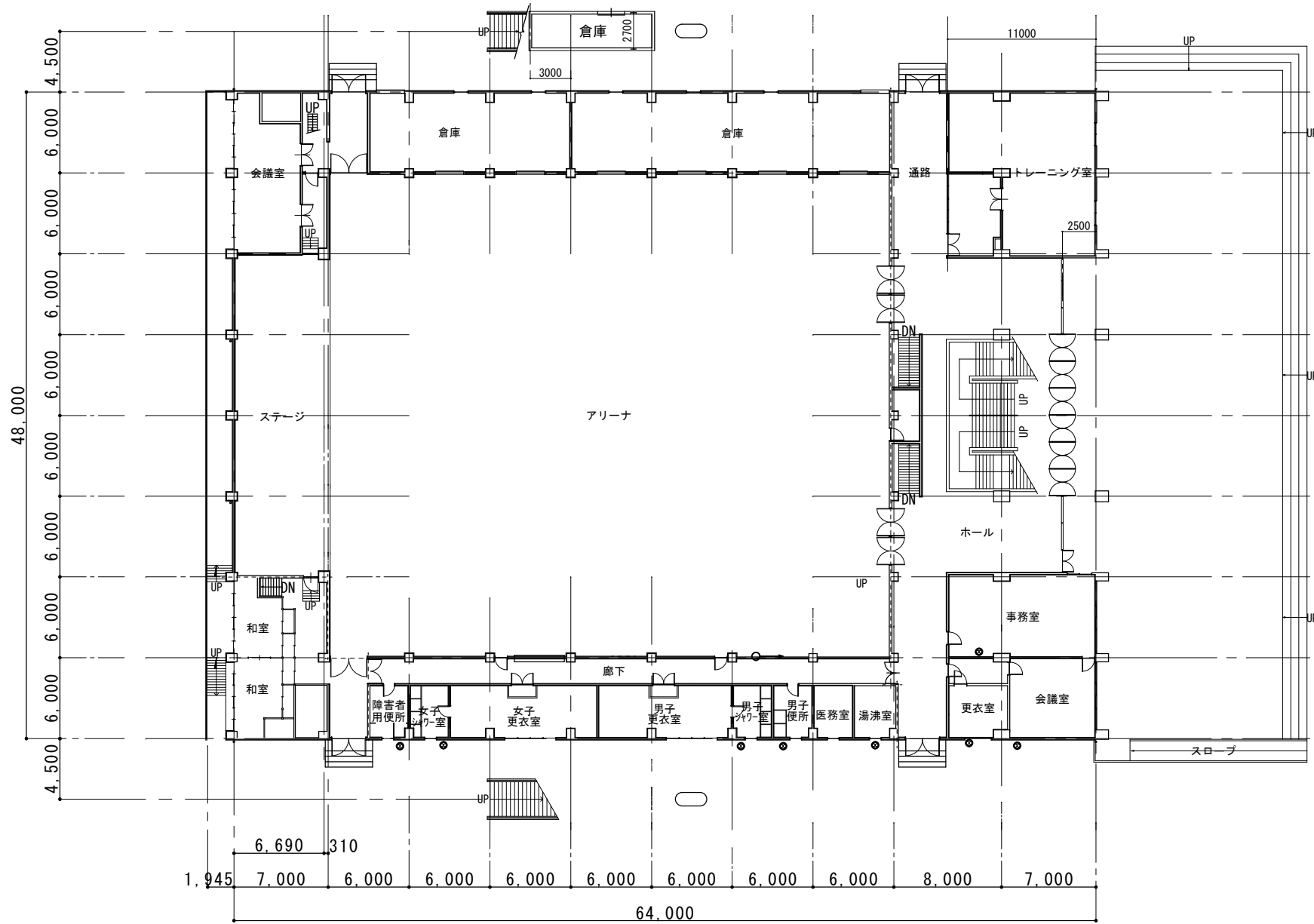
1階平面図
