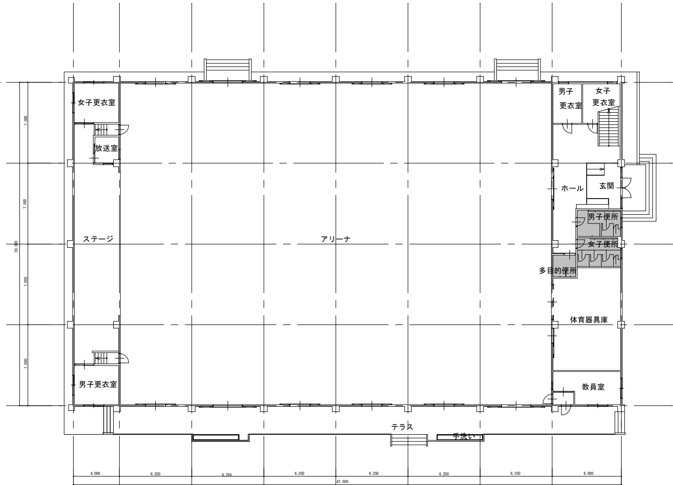
1階平面図
