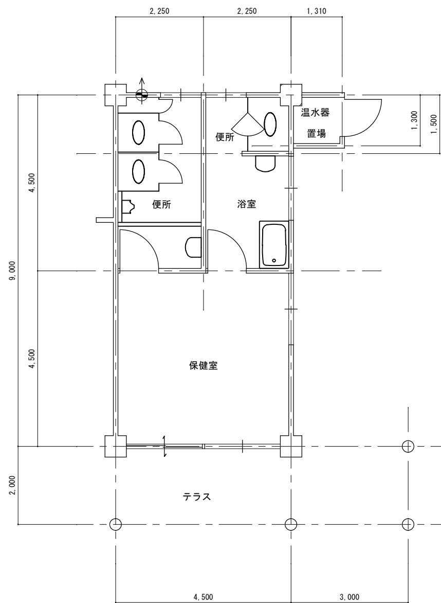
1階平面図
