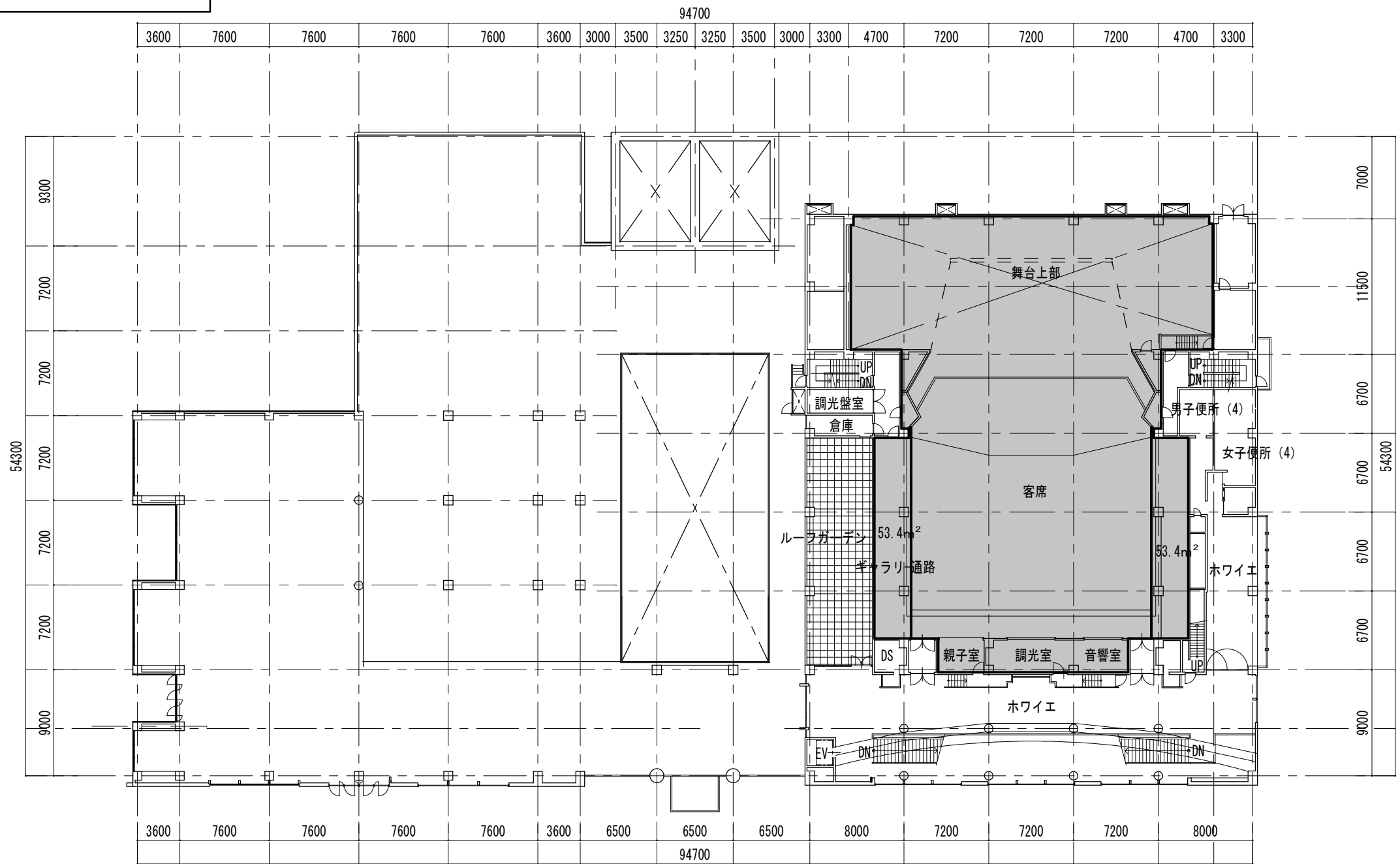
2 階平面図
