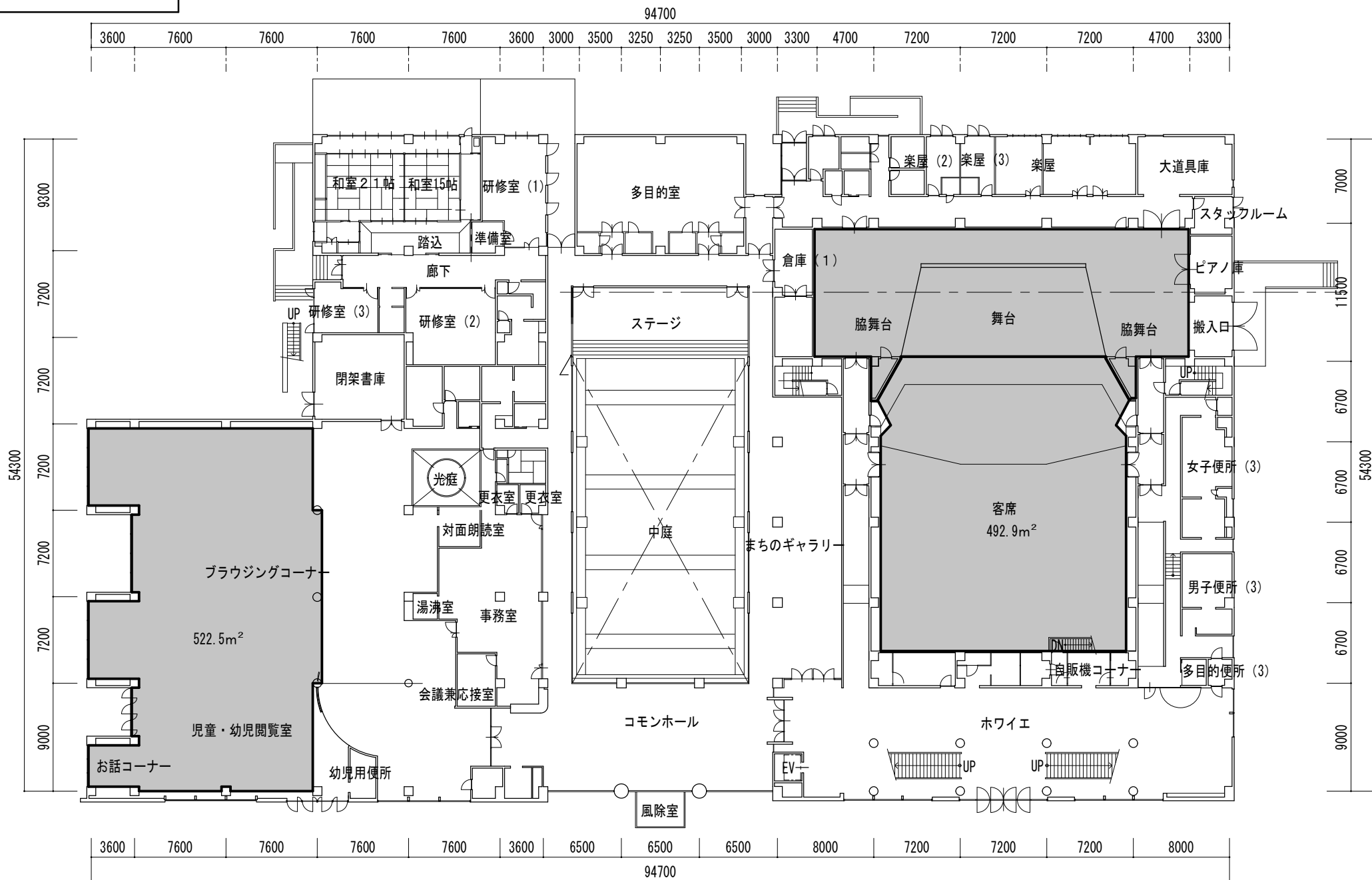
1階平面図
