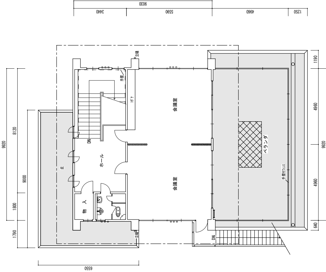
2 階平面図
