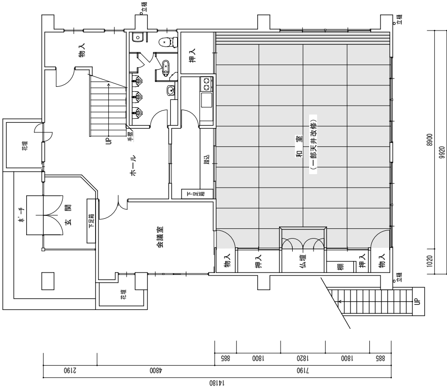
1 階平面図
