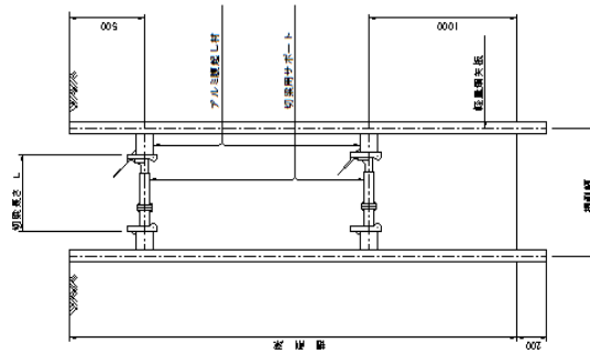
断面図 Sh120
