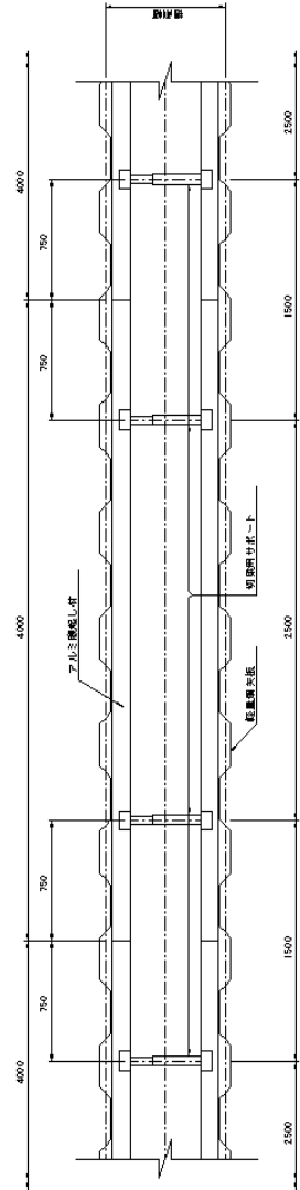
平面図 Sh120
