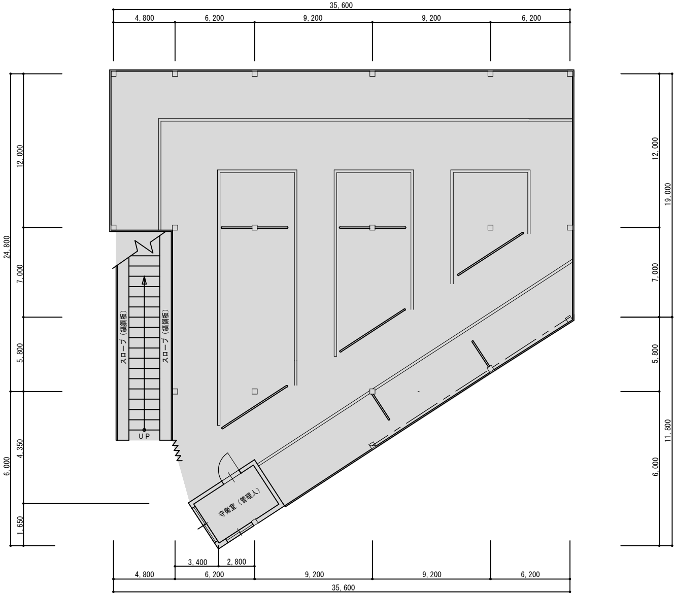
1階平面図
