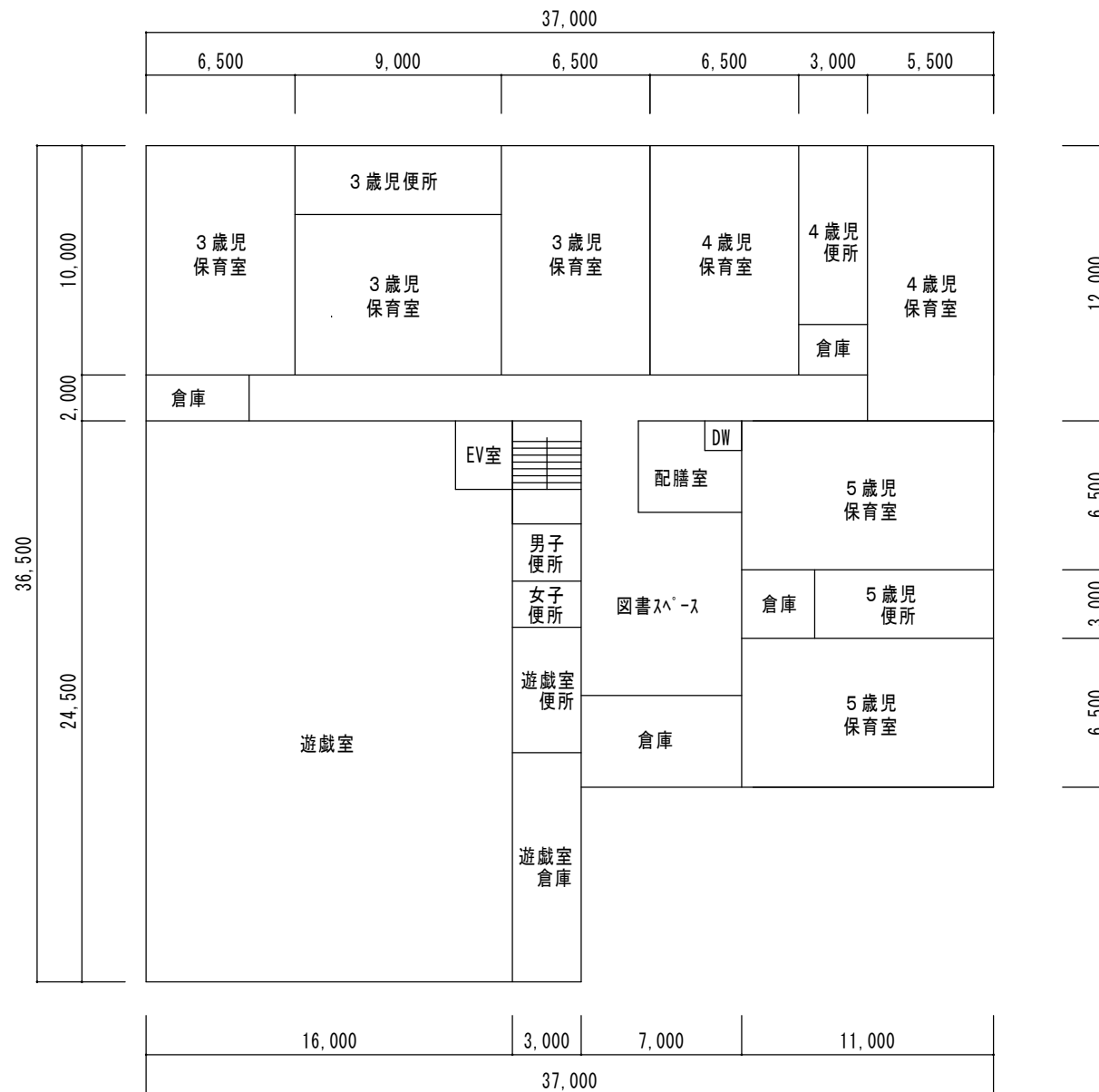
2階平面図 (参考)
