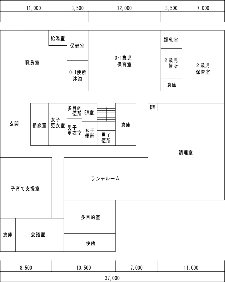
1 階平面図 (参考)
