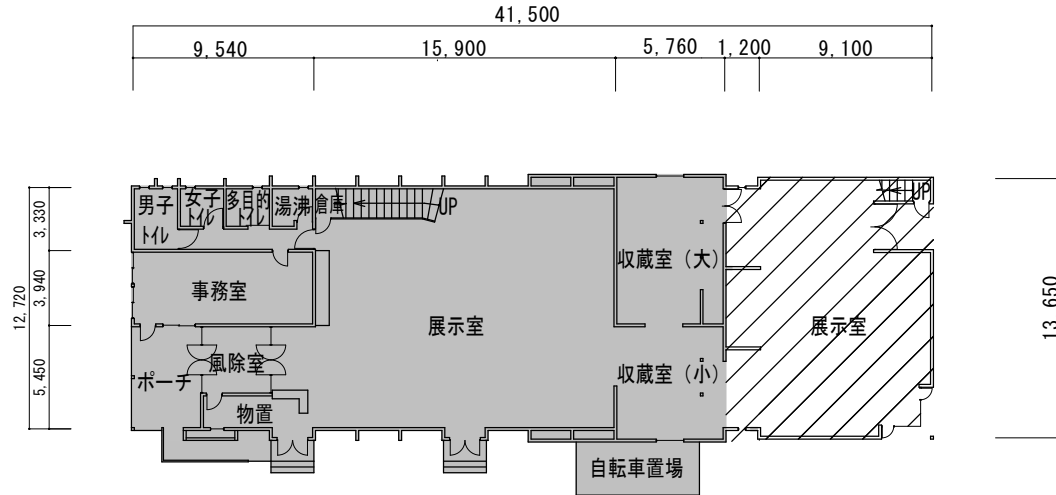
1階平面図
