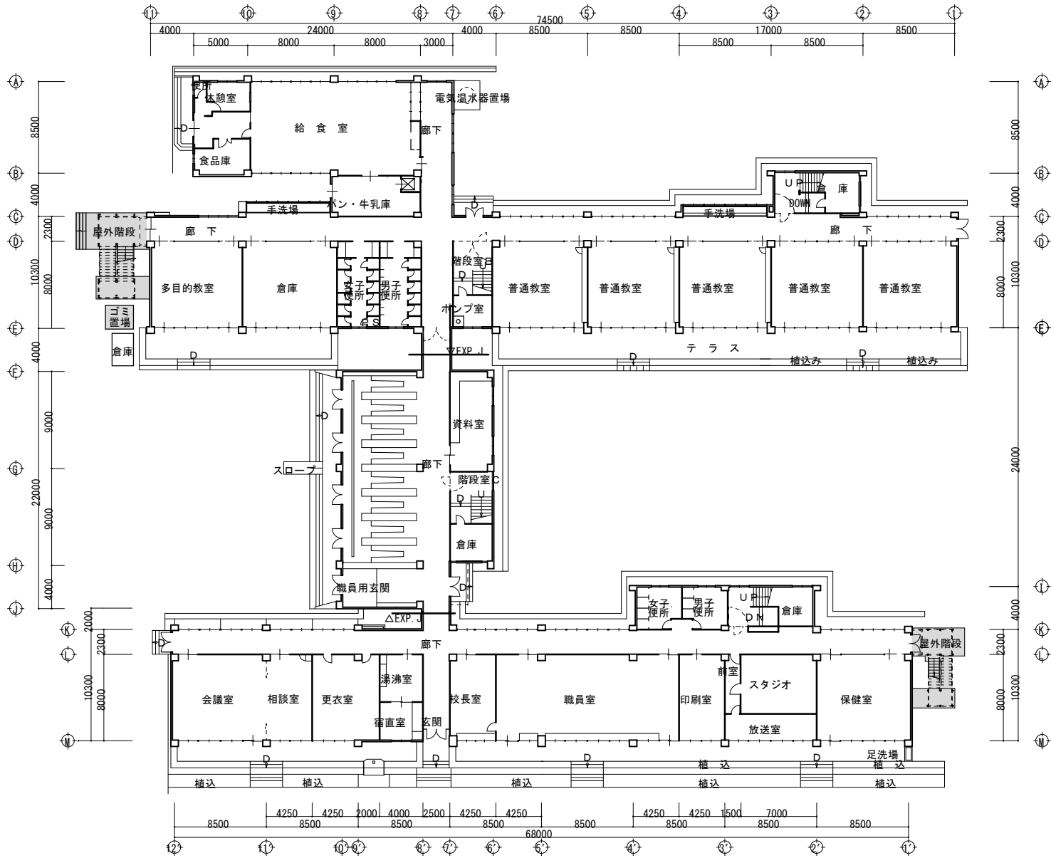
1階平面図
