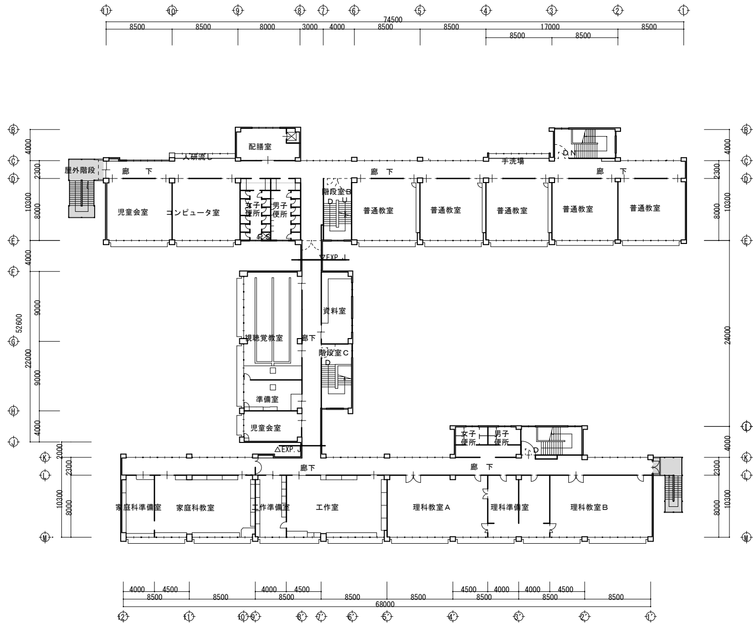
2階平面図
