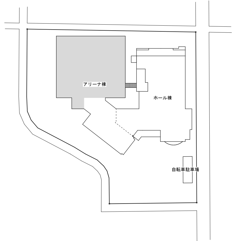
配置図
