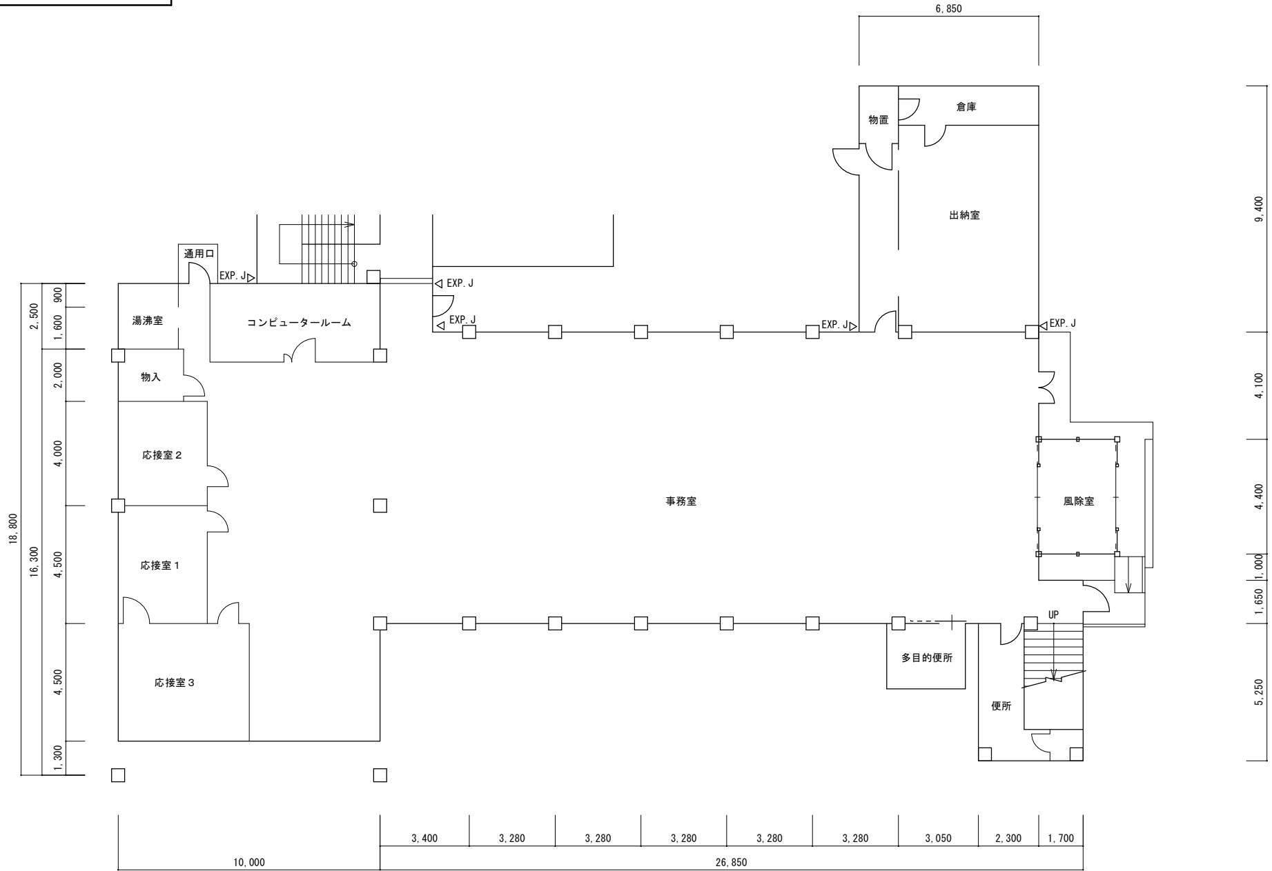
1階平面図
