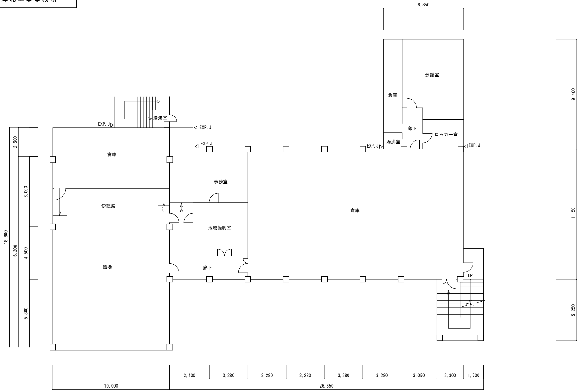
2階平面図
