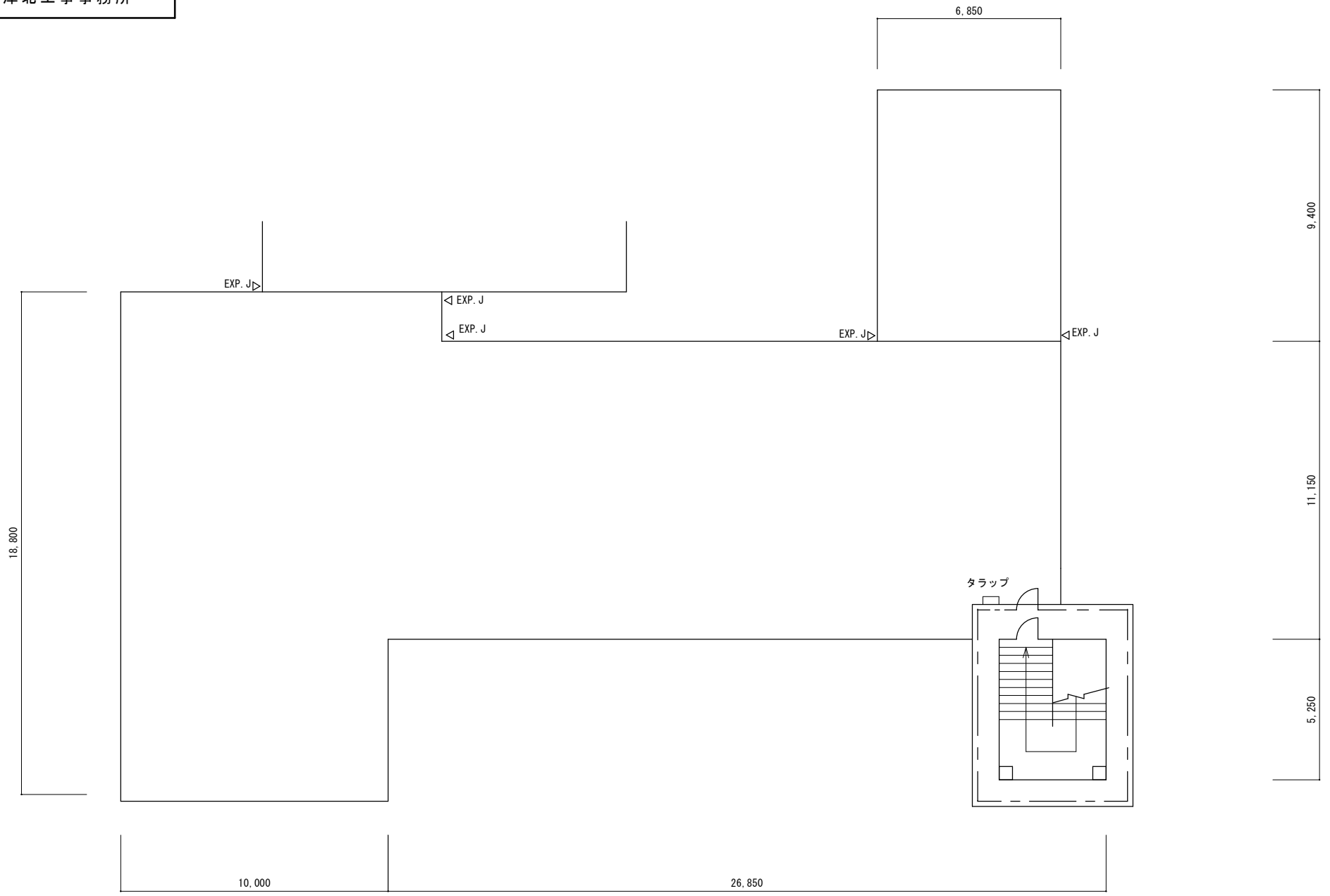
PH階平面図・屋根伏図
