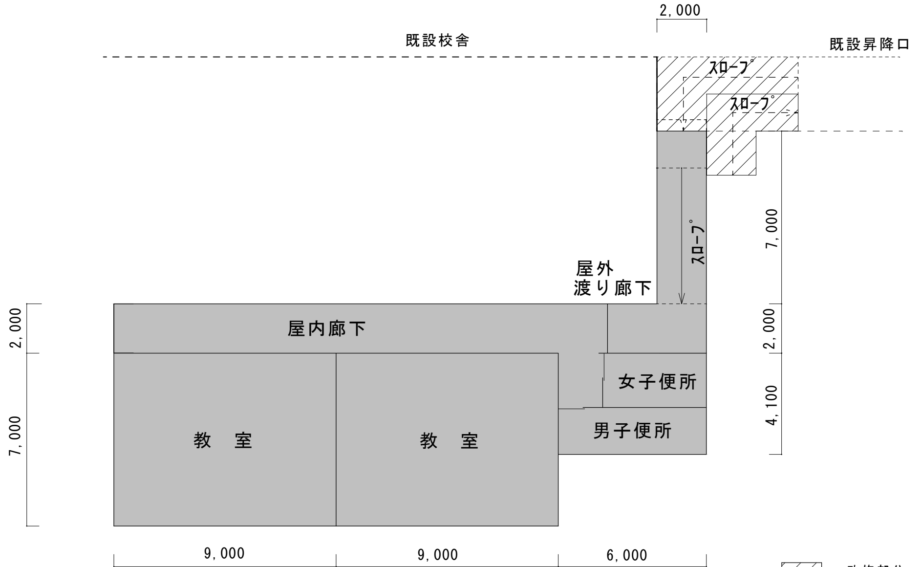
平面図 (参考)
