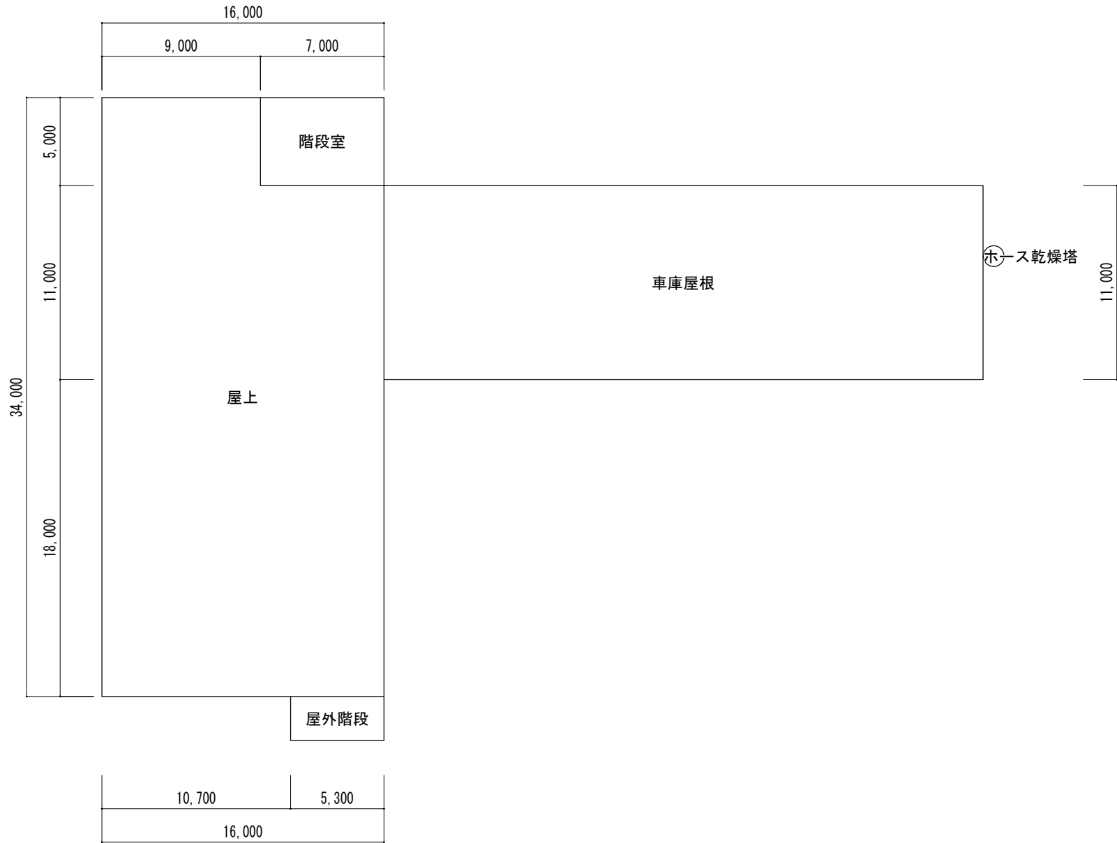
屋上平面図(参考)
