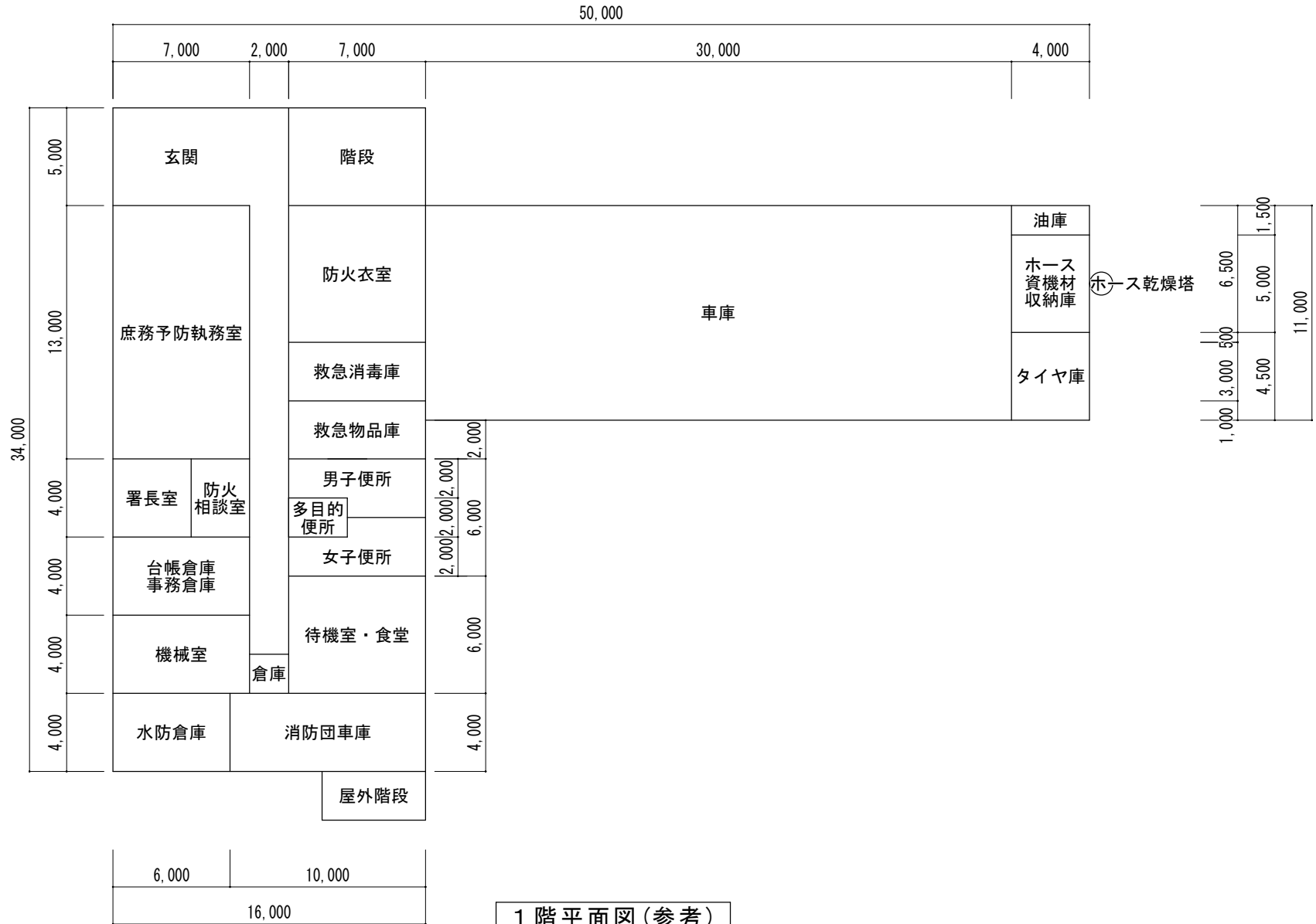
1階平面図(参考)
