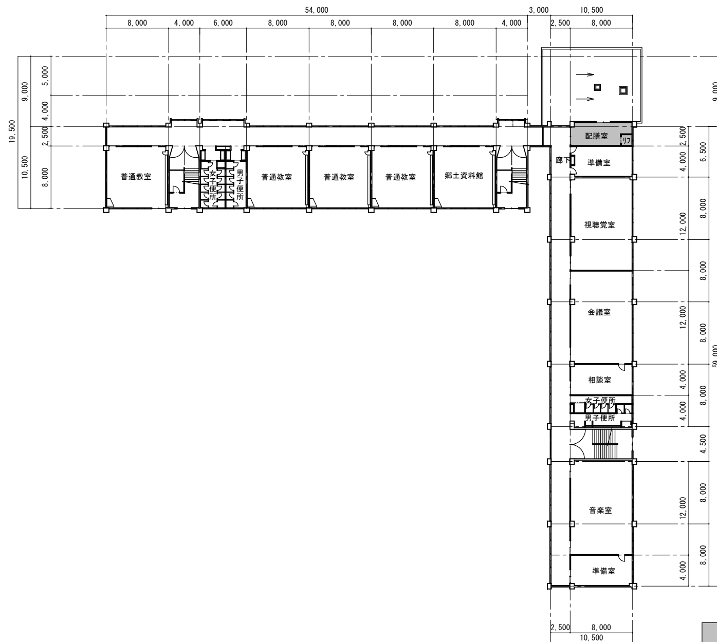
3階平面図
