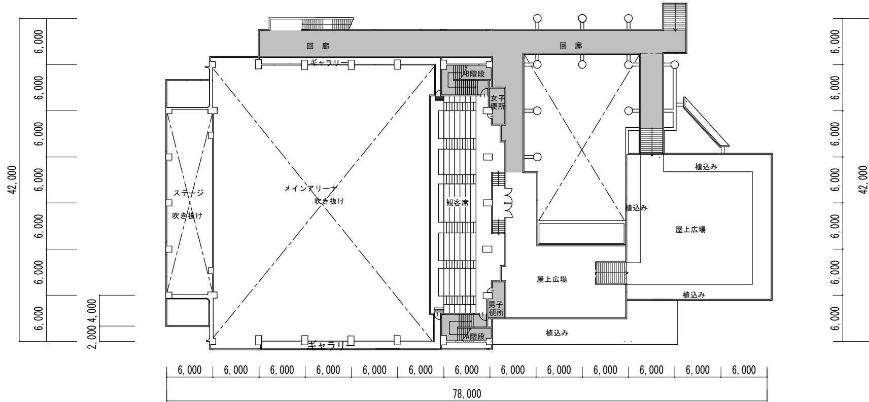
2階平面図
