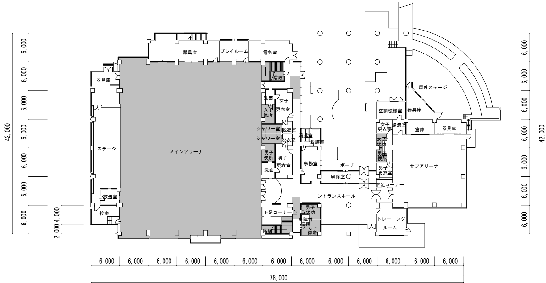
1階平面図
