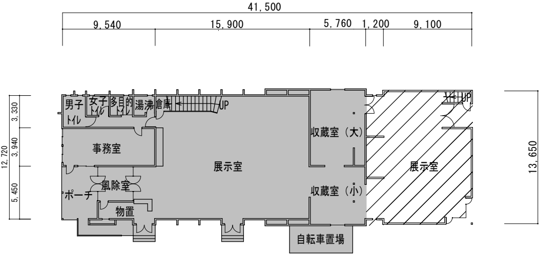
1 階平面図
