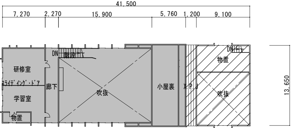
2 階平面図
