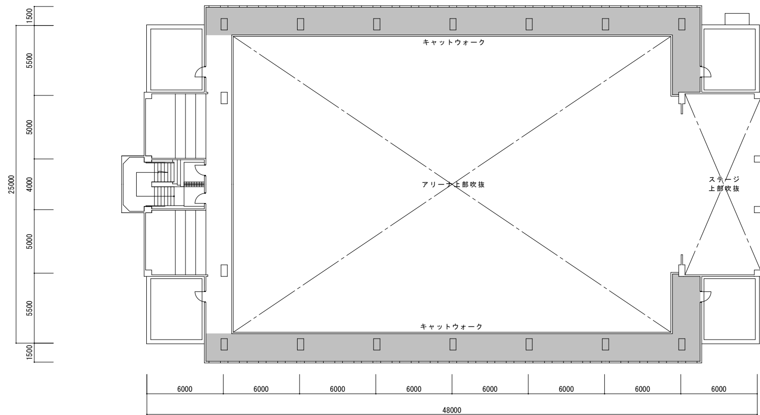
2 階平面図
