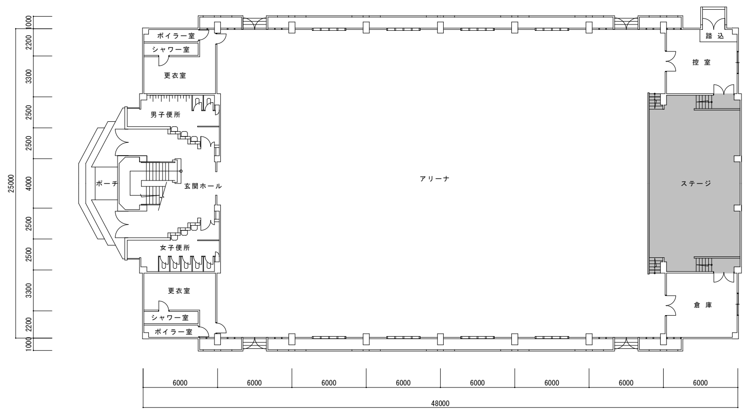
1 階平面図
