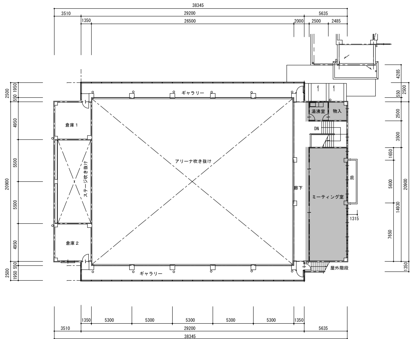
2階平面図
