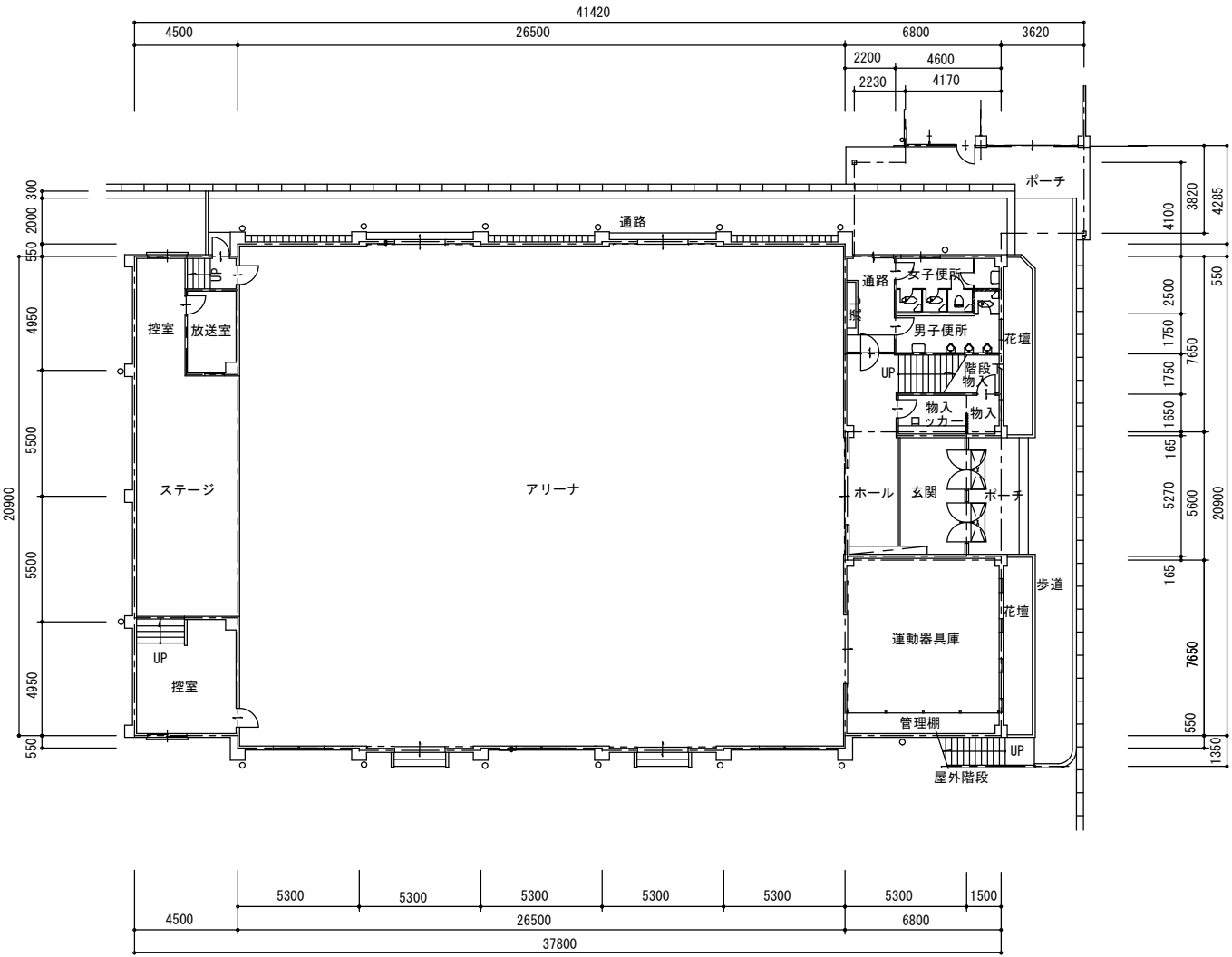
1階平面図
