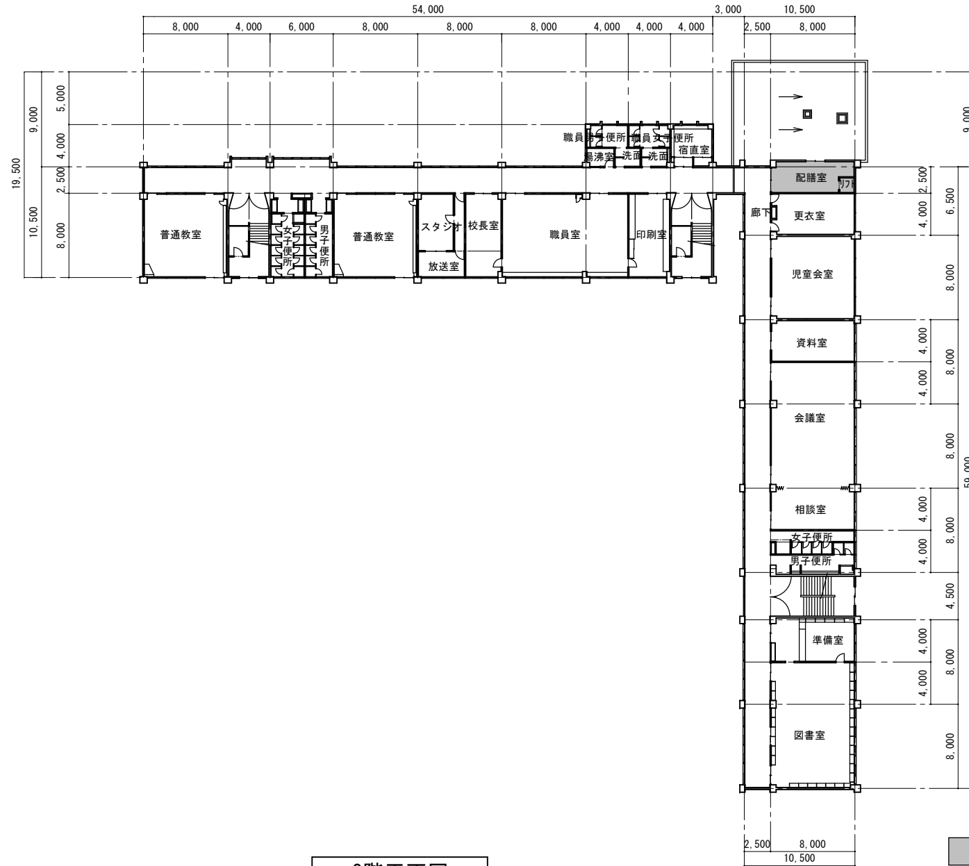
2階平面図
