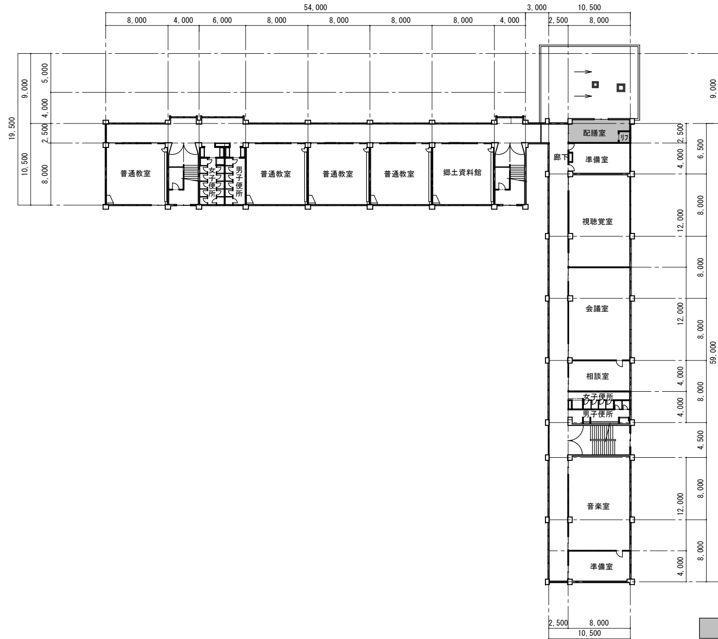
3階平面図
