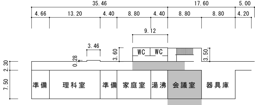
1 階平面図
