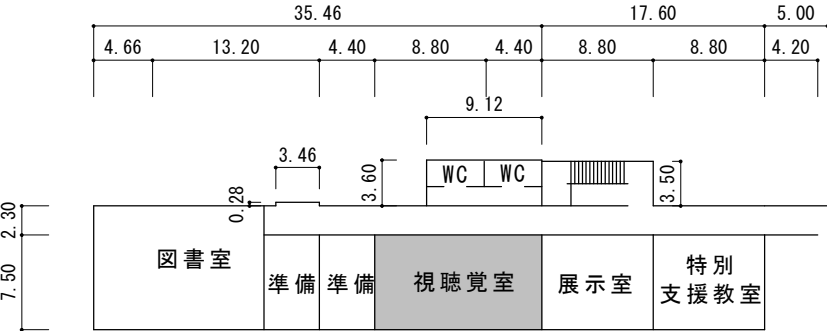
2 階平面図
