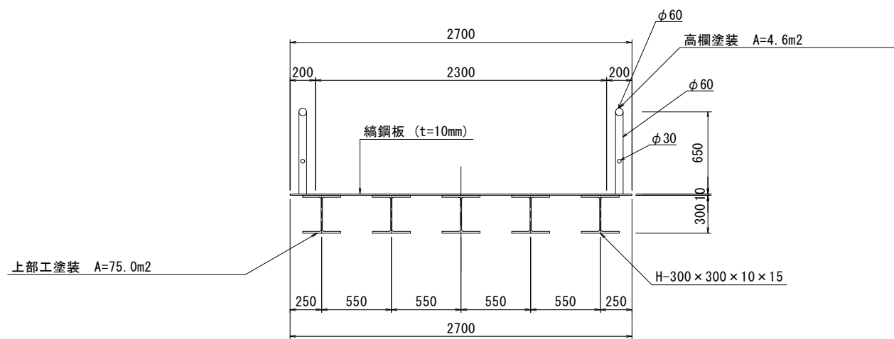
塗装仕様
