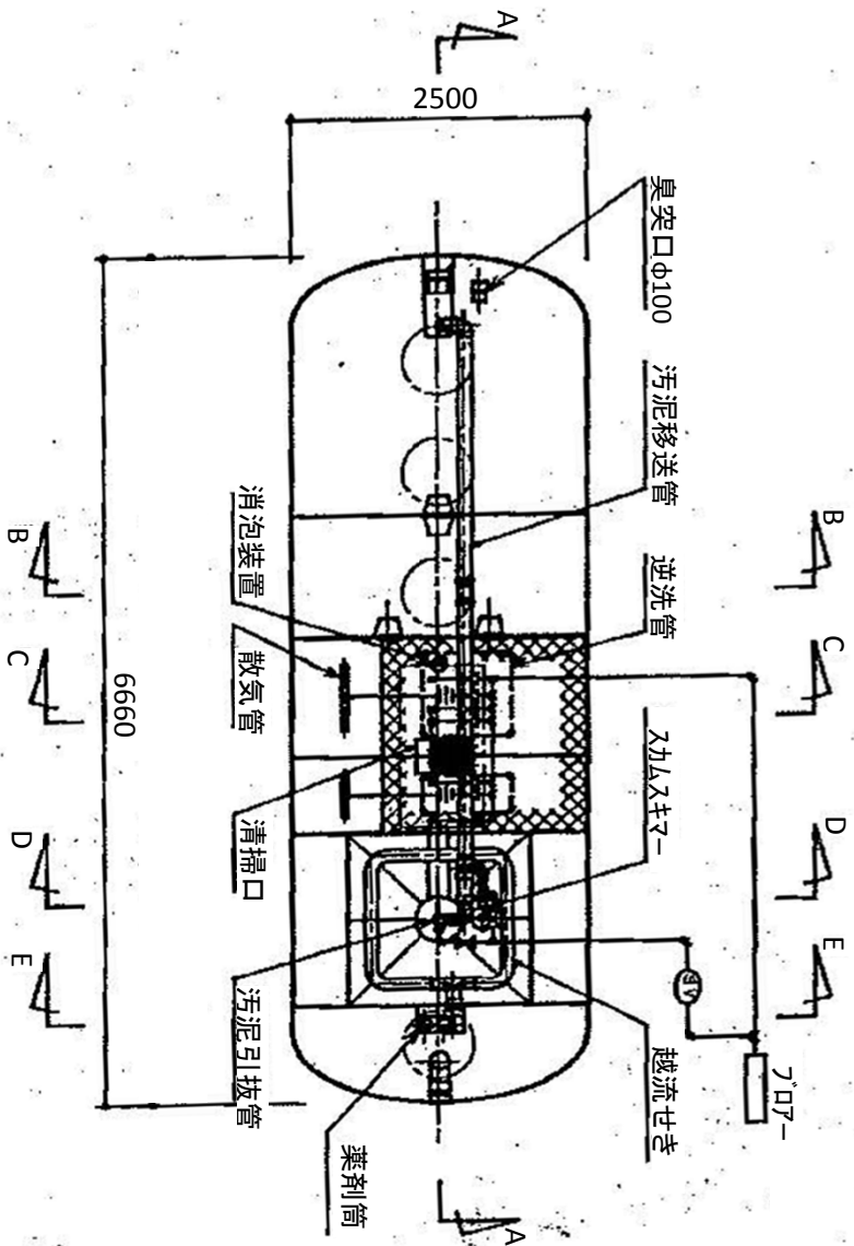
平面図
