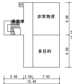
3階
