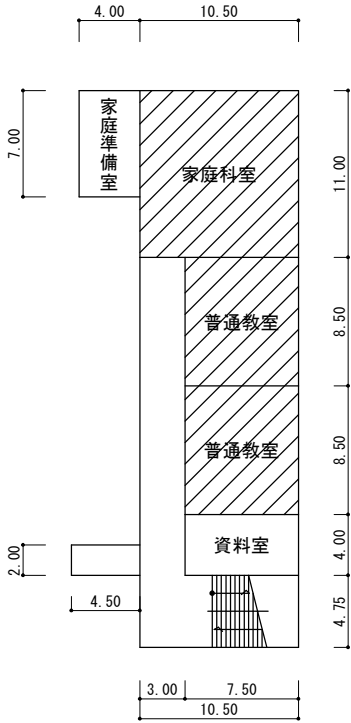
2階
