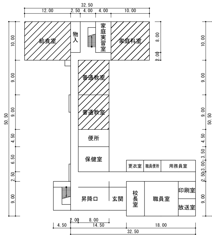
1階
