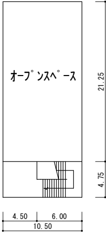
3階
