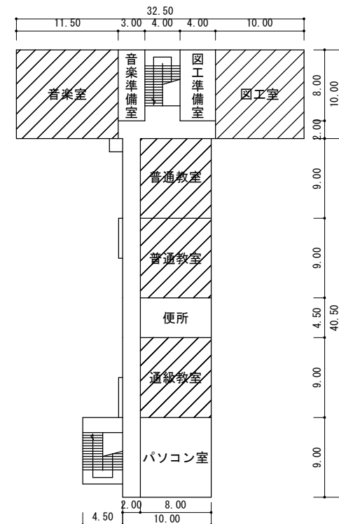
3階
