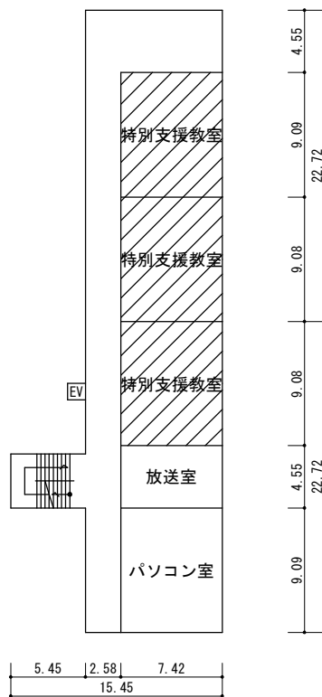
2階
