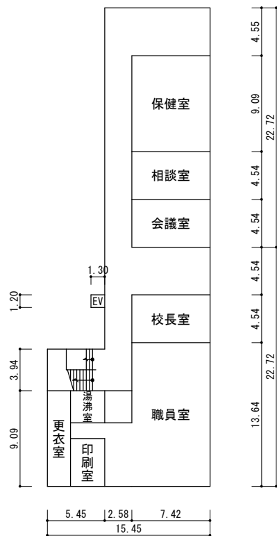
1階
