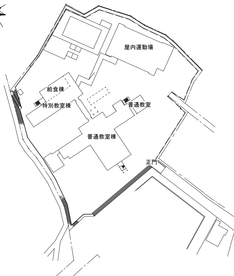
配置図
