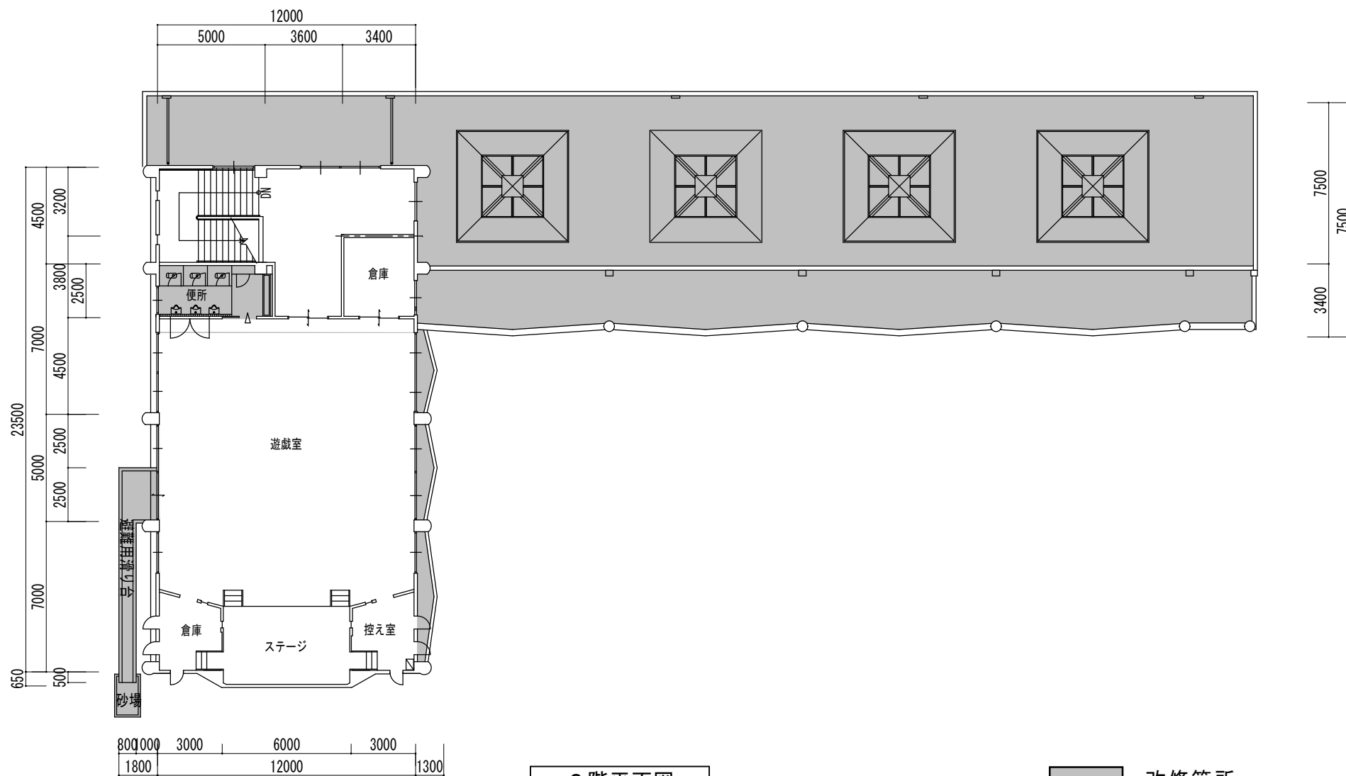
2 階平面図
