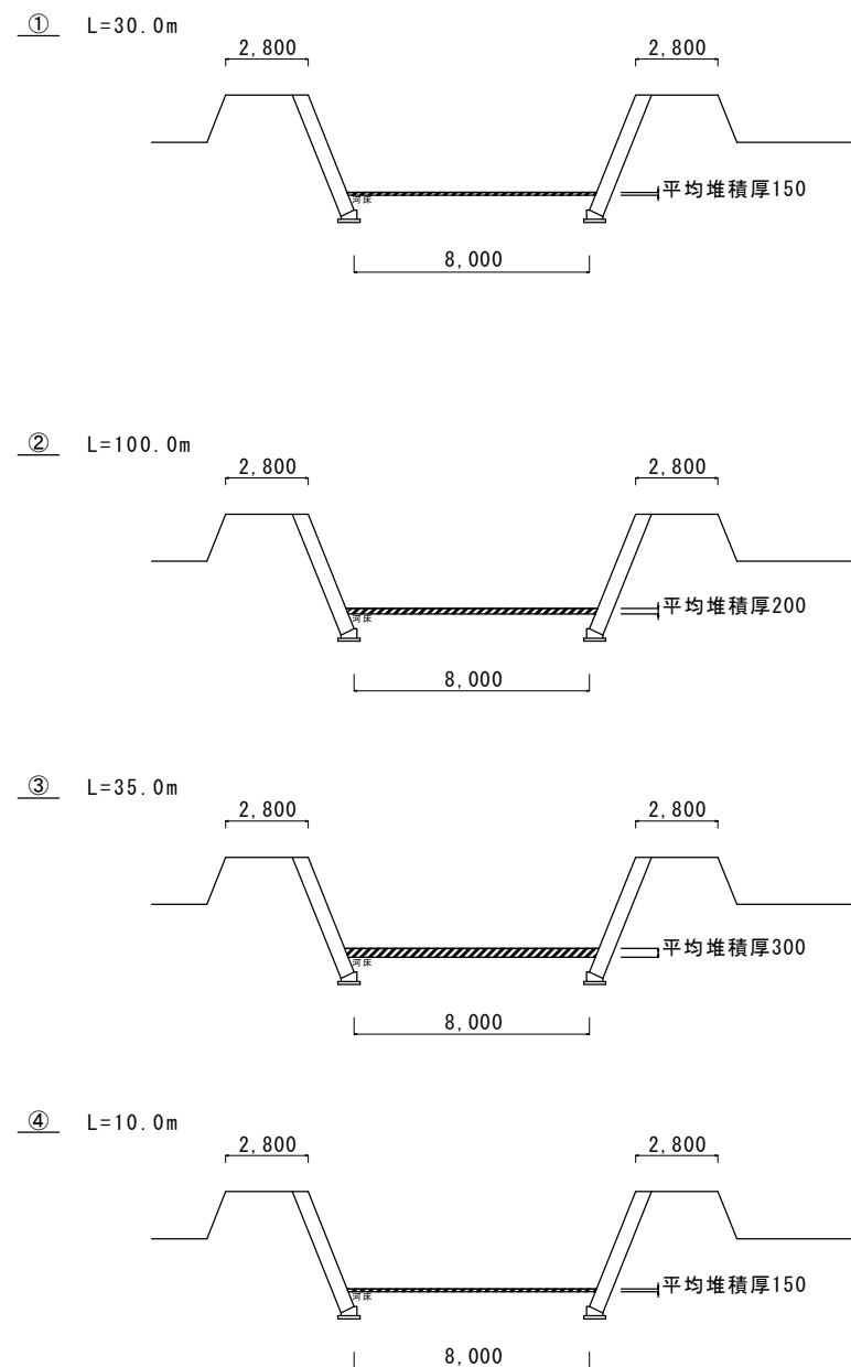
横断面図
