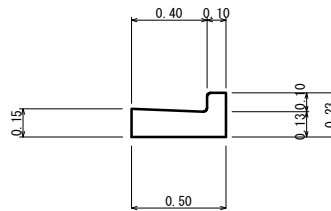
L型側溝 取壊し 10.0m当り
