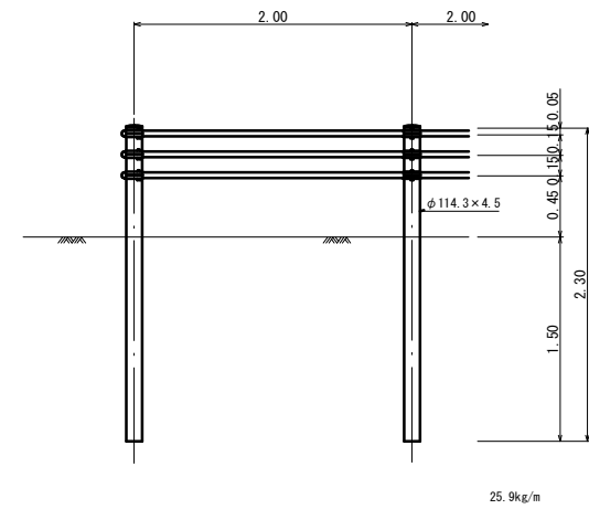
ガードパイプ S=1:40 (Gp-Cp-2E)
