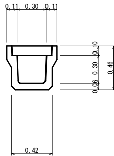
U型側溝 取壊し 10.0m当り
