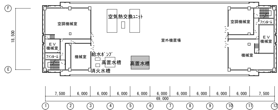
R階平面図
