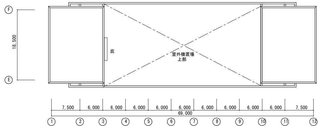
PH階平面図
