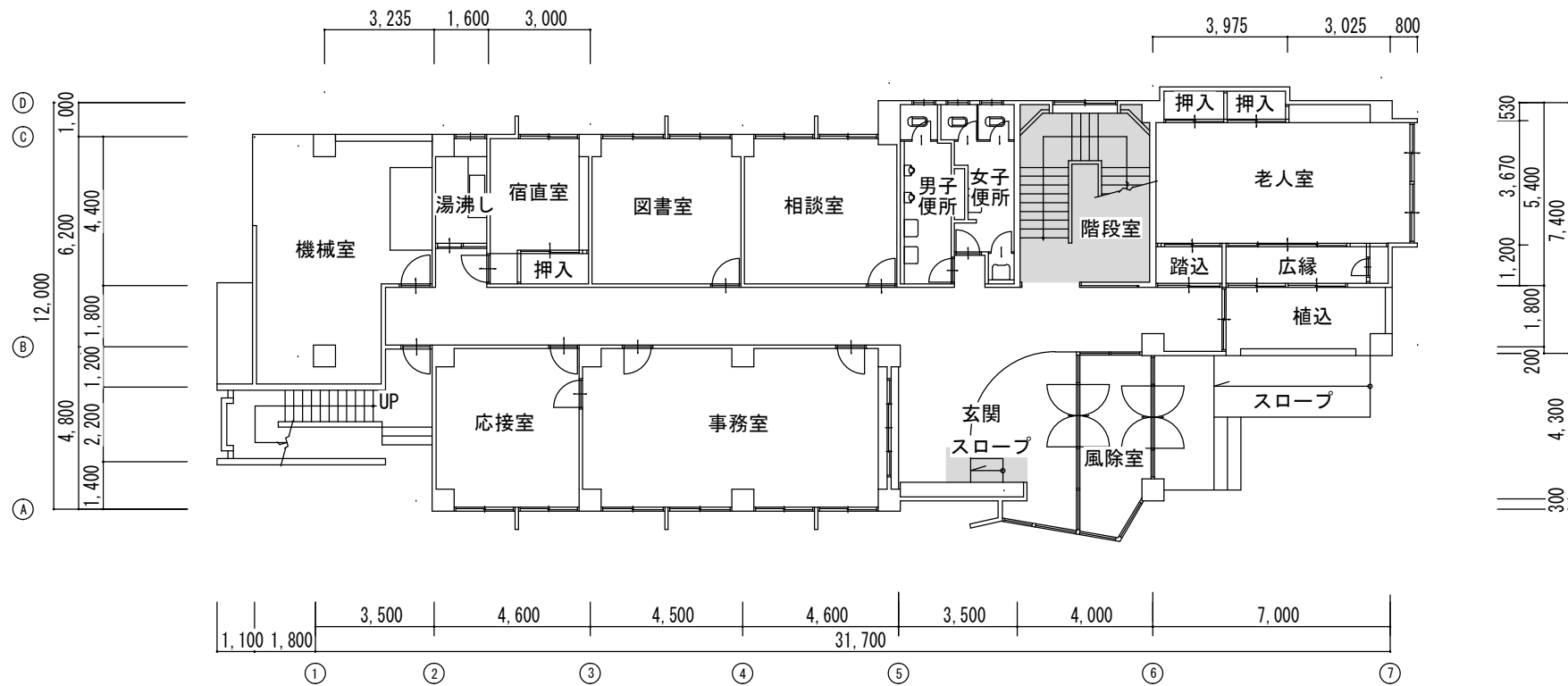
1 階平面図
