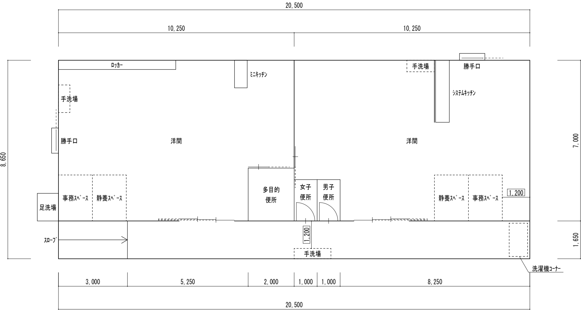
平面図（参考）
