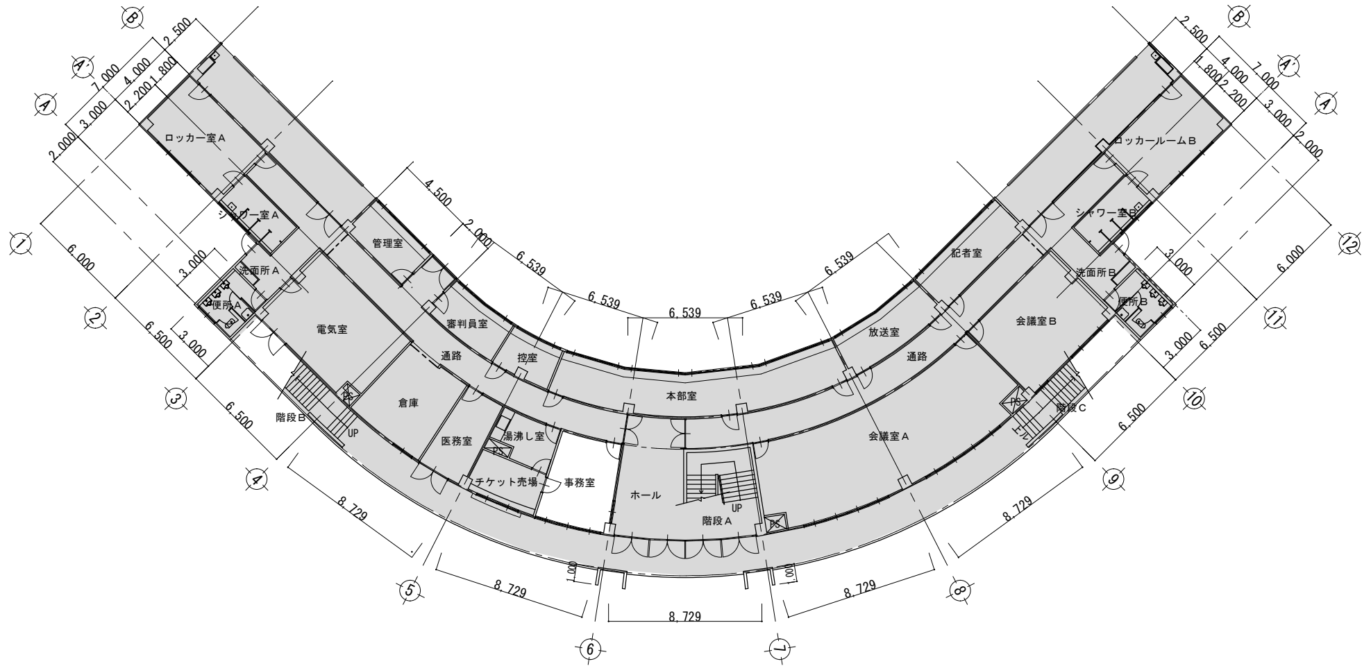
1階平面図
