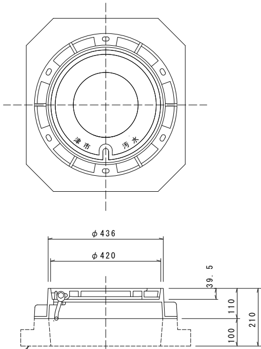
保護鉄蓋 φ300 T-14
