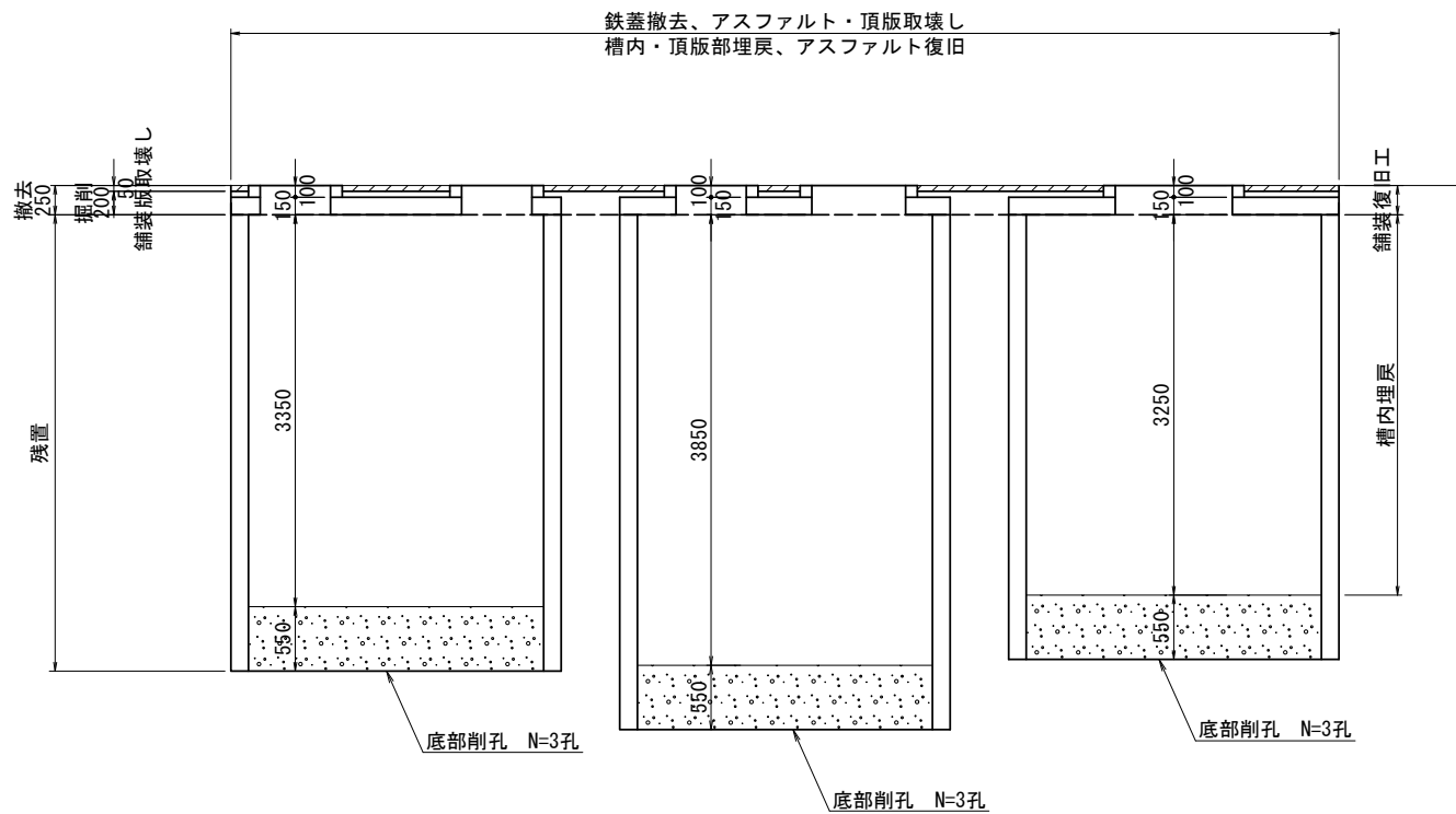
A-A 断面図
