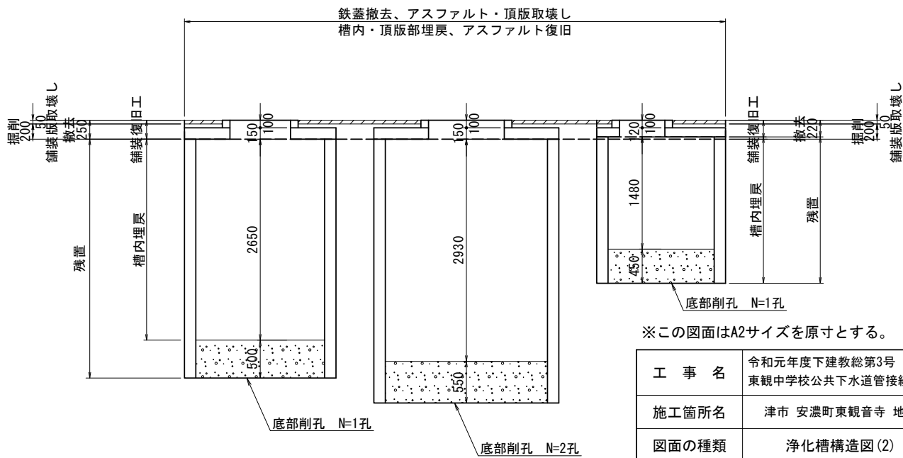
B-B 断面図
