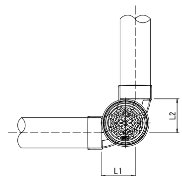
塩ビ製枡
