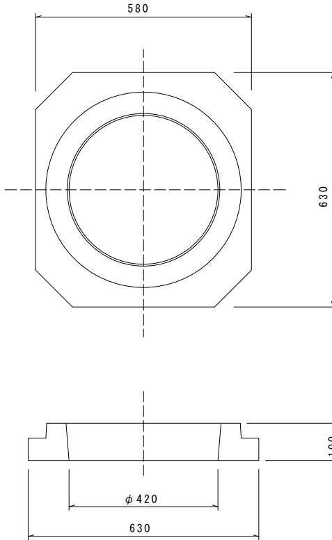
沈下防止板
