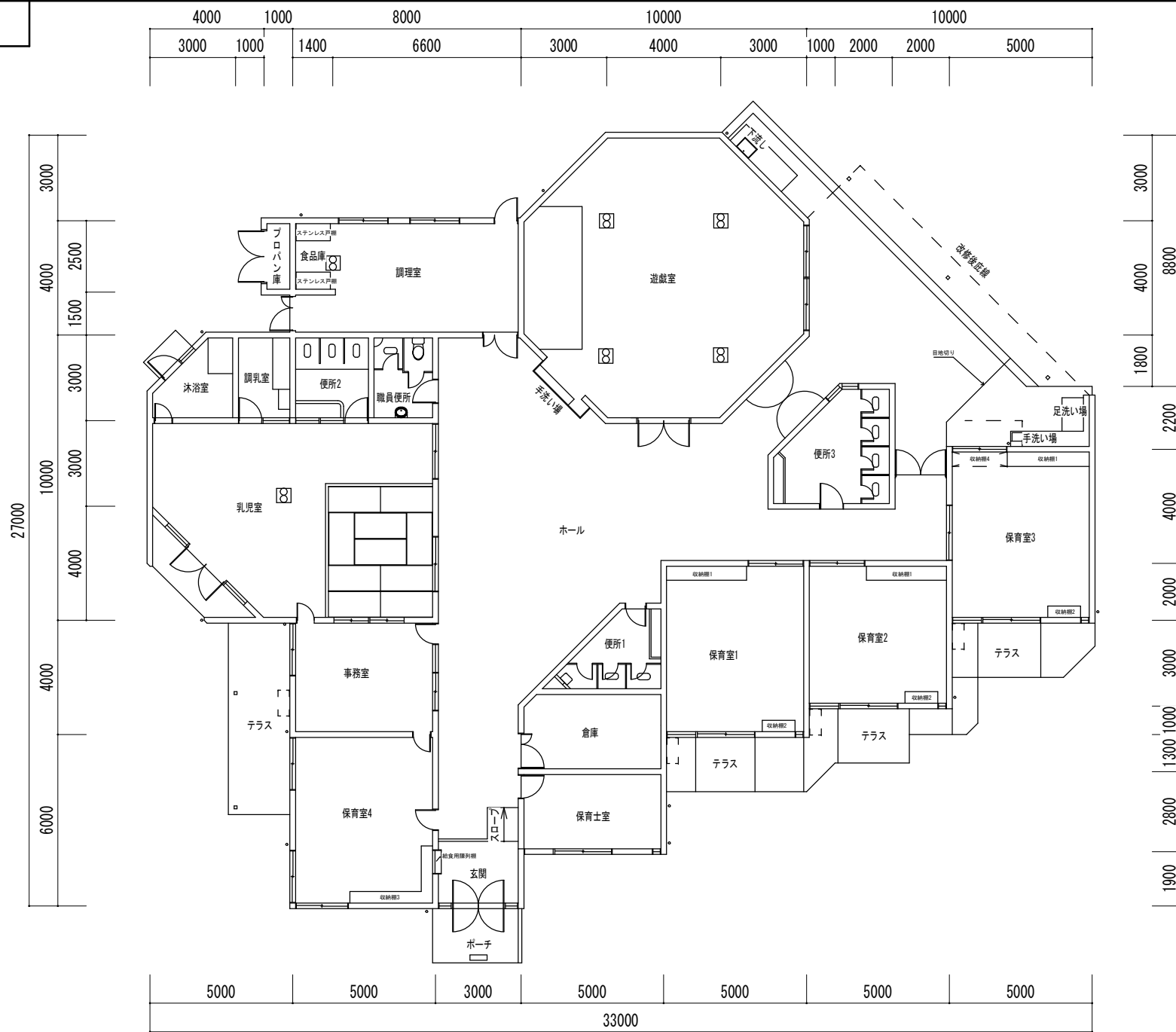
1階平面図
