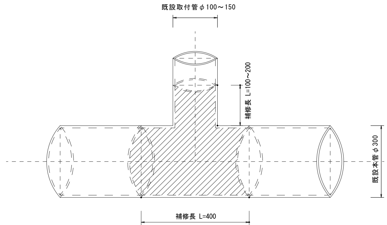
支管一体部分補修工
