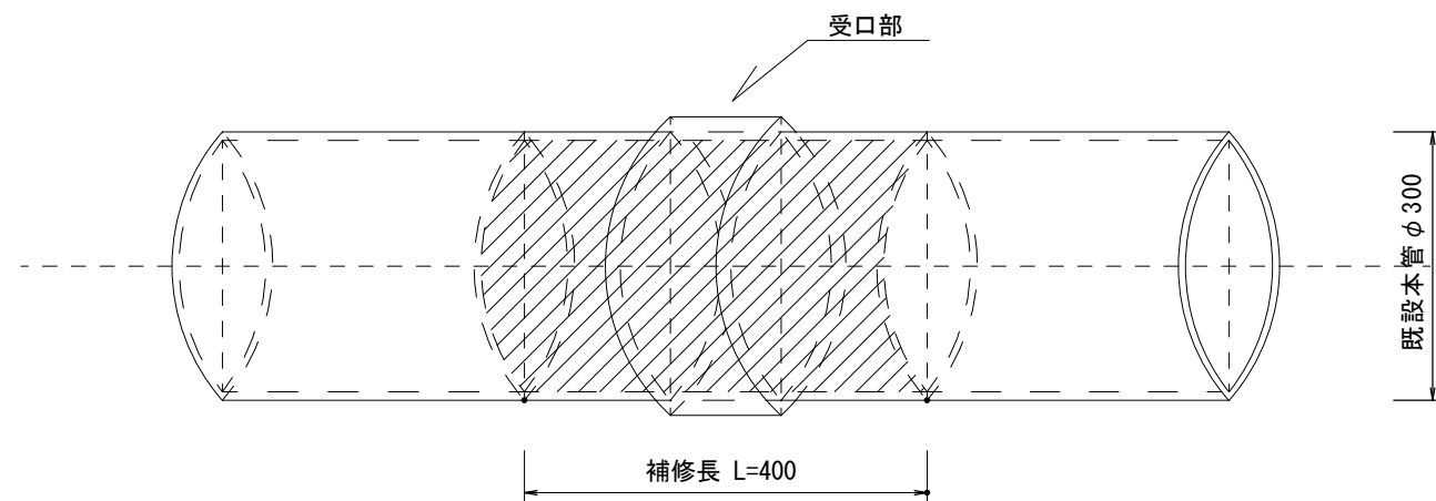
本管部分補修工
