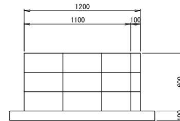
B-B断面図
