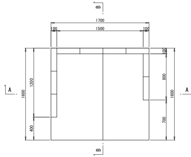
平面図
