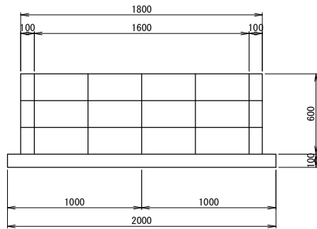
A-A断面図
